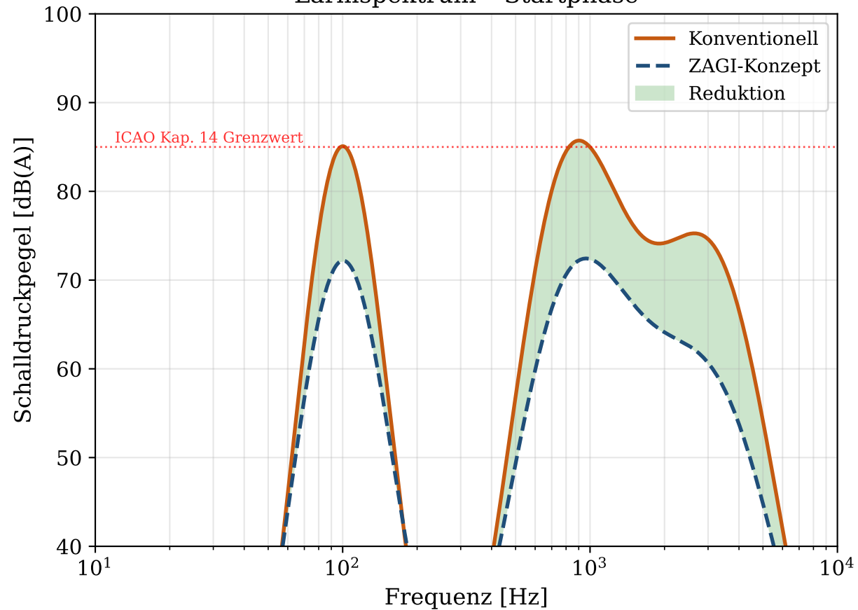
Lärmspektrum - Startphase
