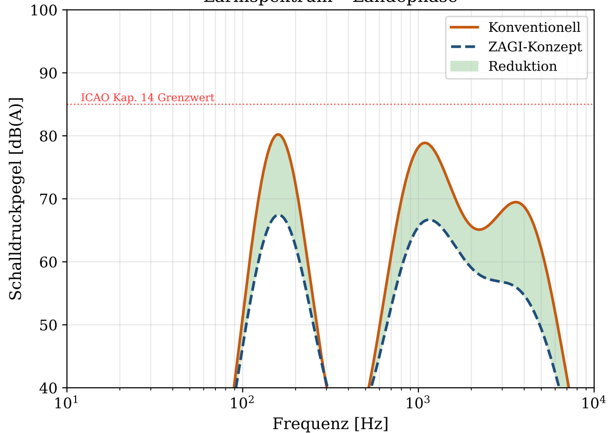
Lärmspektrum - Landephase
