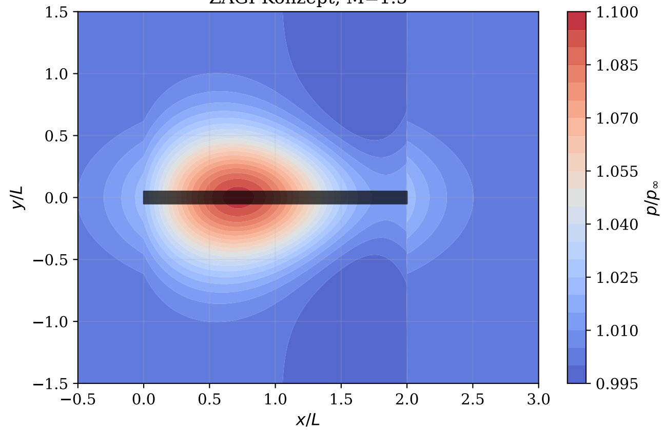
ZAGI-Konzept, M=1.5
