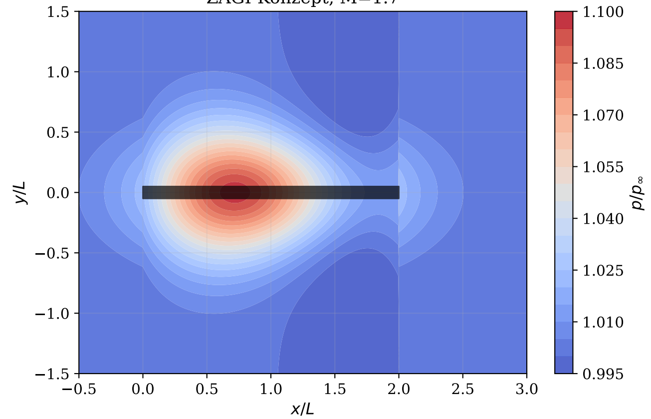
ZAGI-Konzept, M=1.7
