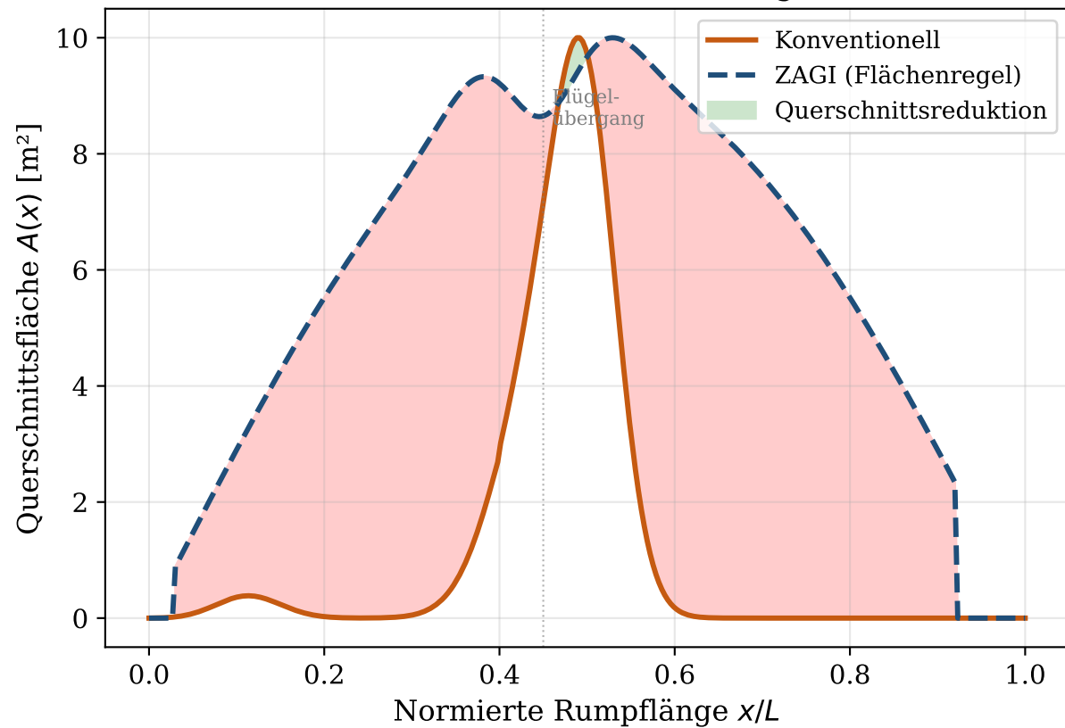
Querschnittsverlauf A(x) entlang der Rumpfachse - Whitcombsche Flächenregel
