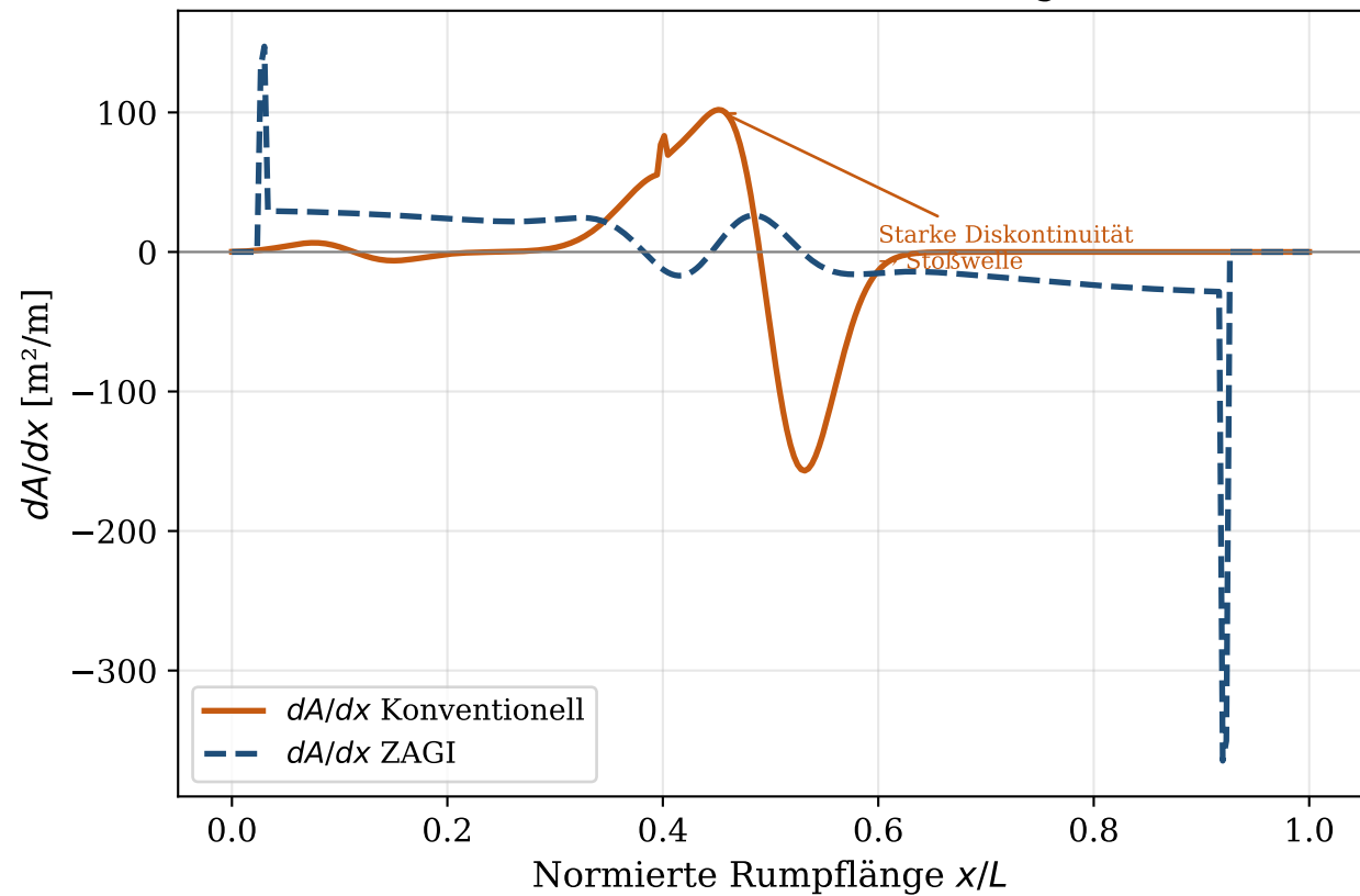
Ableitung des Querschnittsverlaufs dA/dx - Kriterium für Wellenbildung
