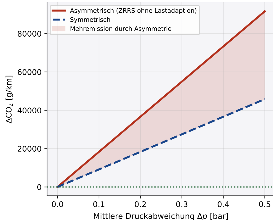
CO 2 -Mehremission durch asymm. Druck
