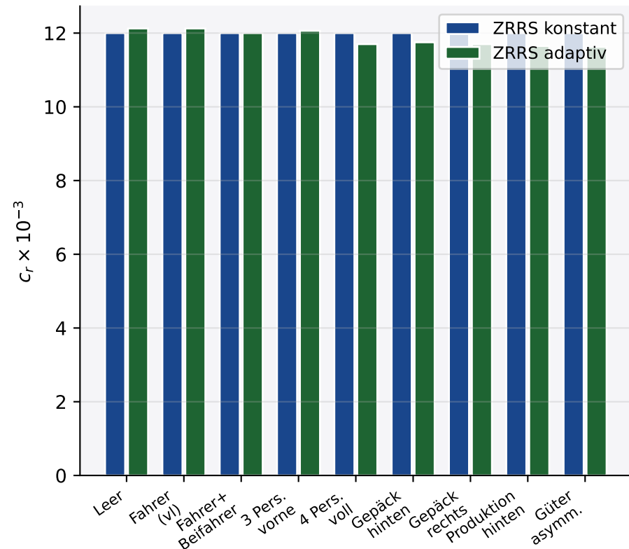
Rollwiderstand pro Szenario
