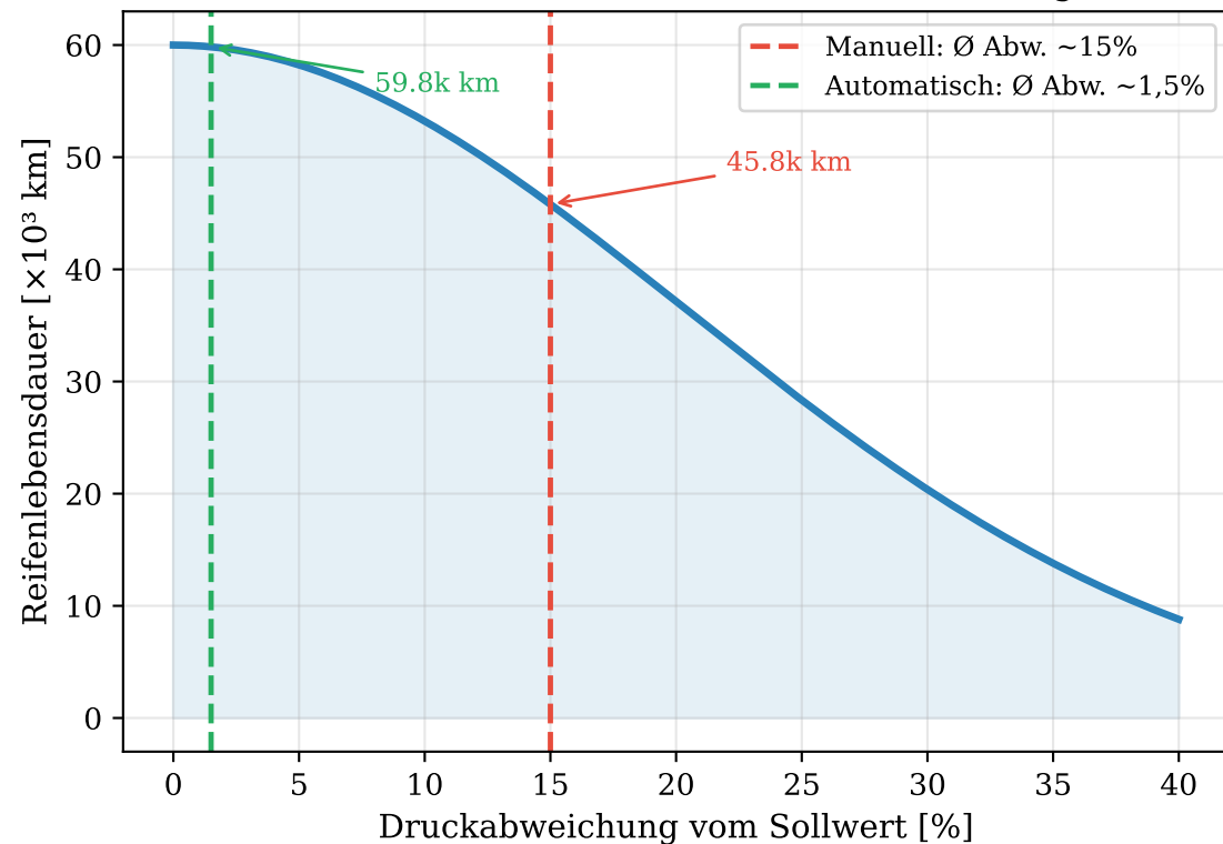
(a) Reifenlebensdauer vs. Druckabweichung
