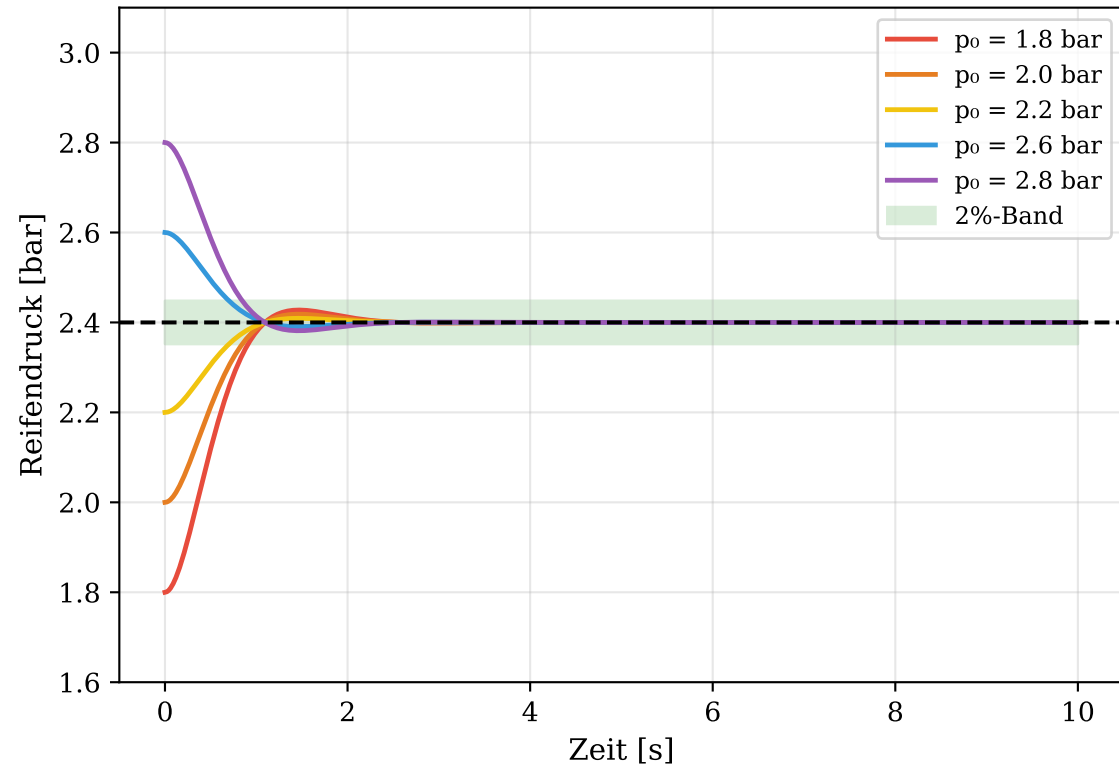
(a) Sprungantworten des Druckregelkreises (verschiedene Anfangsdrücke)
