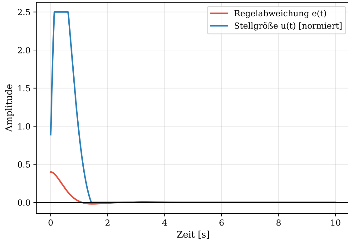
(b) Regelabweichung und Stellgröße (Startdruck 2,0 bar \rightarrow Sollwert 2,4 bar)
