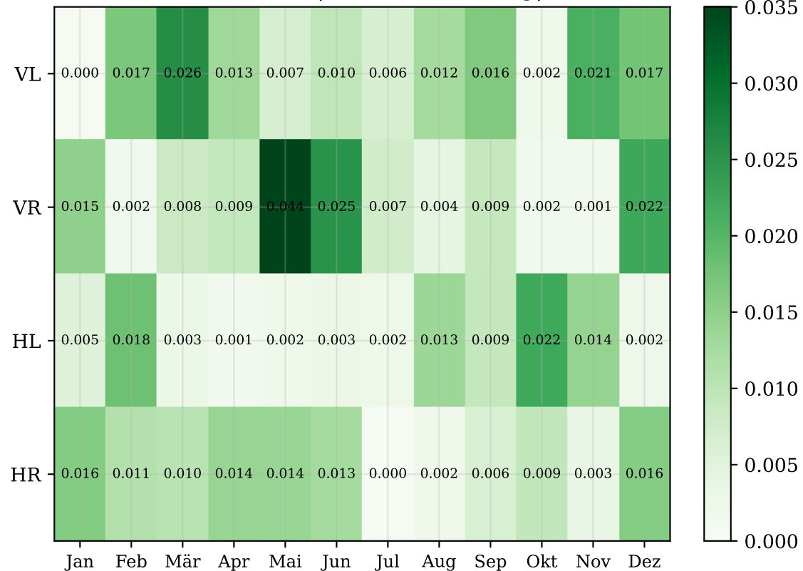
(b) Automatisch: |Druckabweichung| [bar]
