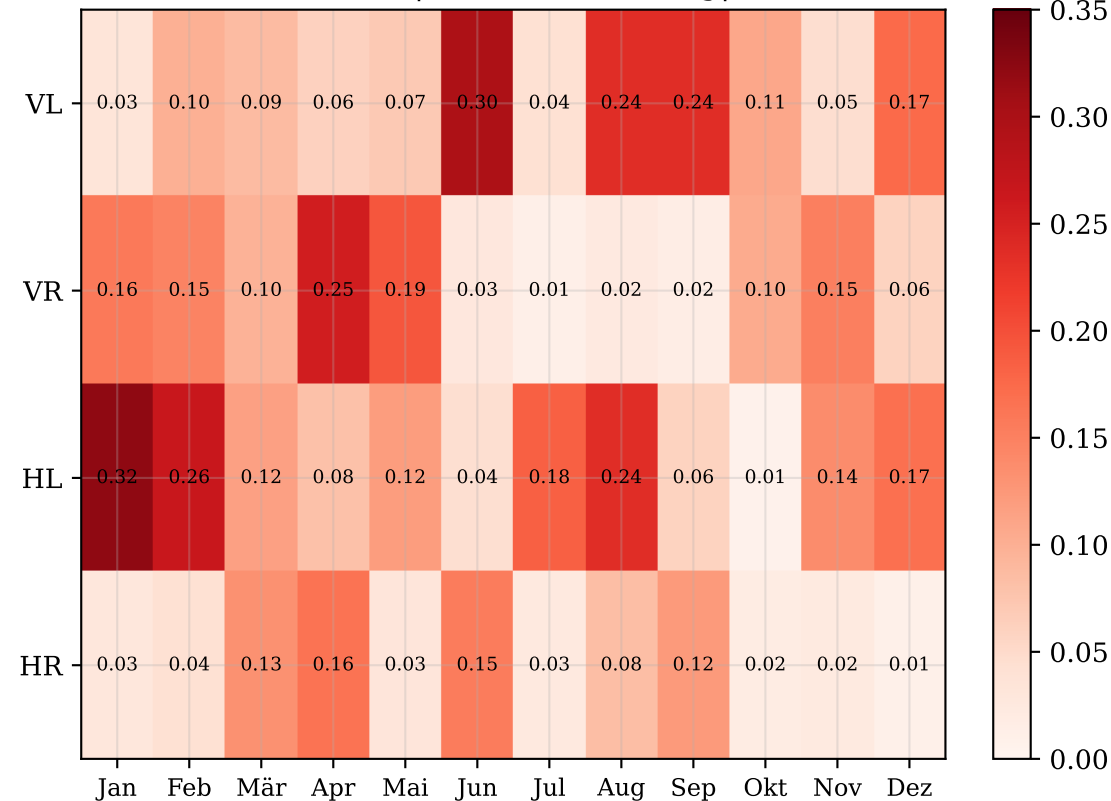
(a) Manuell: |Druckabweichung| [bar]
