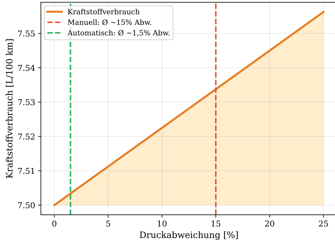
(a) Kraftstoffverbrauch vs. Druckabweichung
