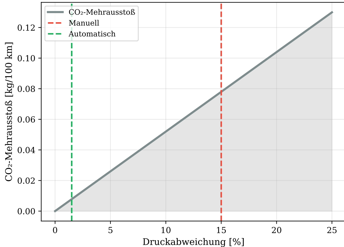
(b) CO 2 -Mehrausstoß vs. Druckabweichung
