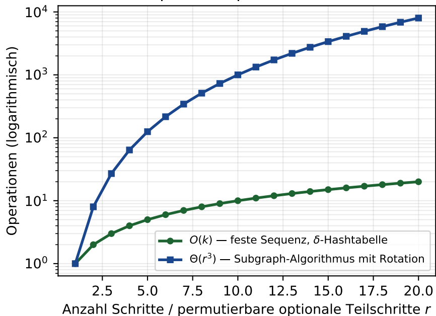
Konformitätsprüfung: lineare Sequenz vs. permutierbare Schritte
