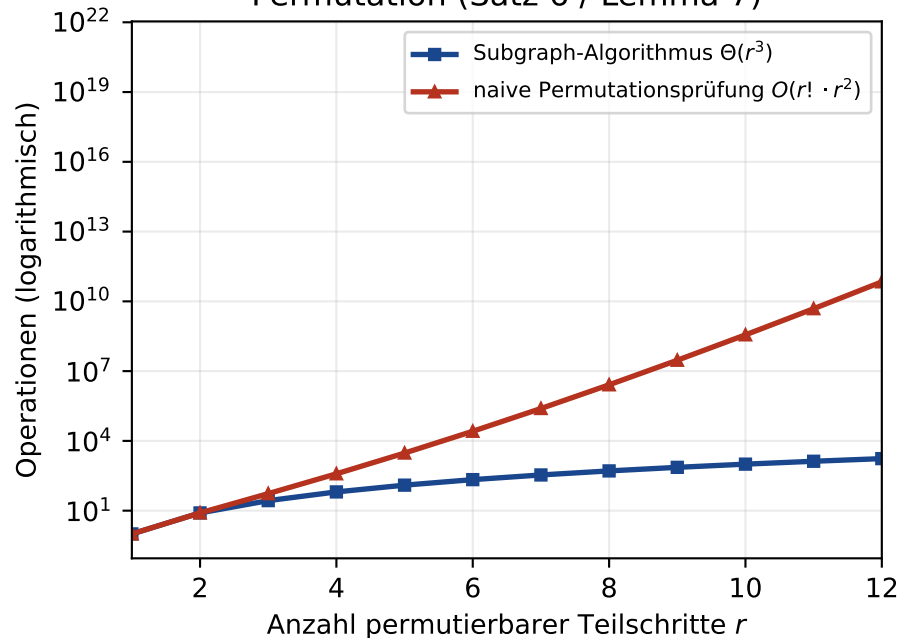
Rotation vs. vollständige Permutation (Satz 6 / Lemma 7)
