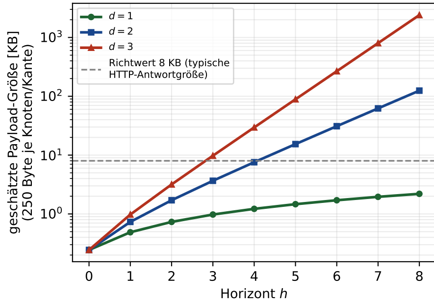
Übertragungsaufwand des Horizont-Subgraphen G_s^h
