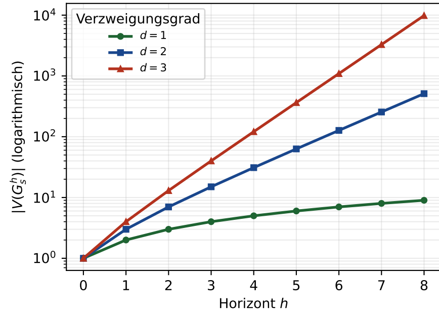
Größe des Horizont-Subgraphen nach Lemma 2 (Abschnitt 7.4)
