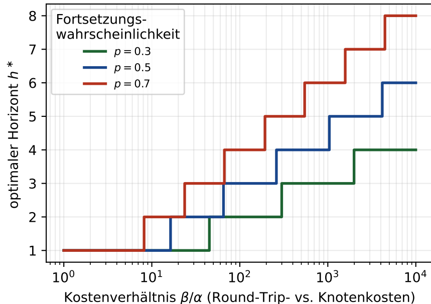
Optimaler Horizont h^* in Abhängigkeit von \beta/\alpha ( d = 2 )
