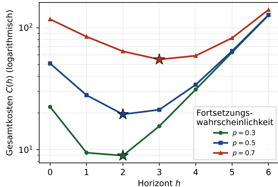
Kostenfunktion C(h) und optimaler Horizont h^* (Satz 6, \alpha = 1, \beta = 50, d = 2 )
