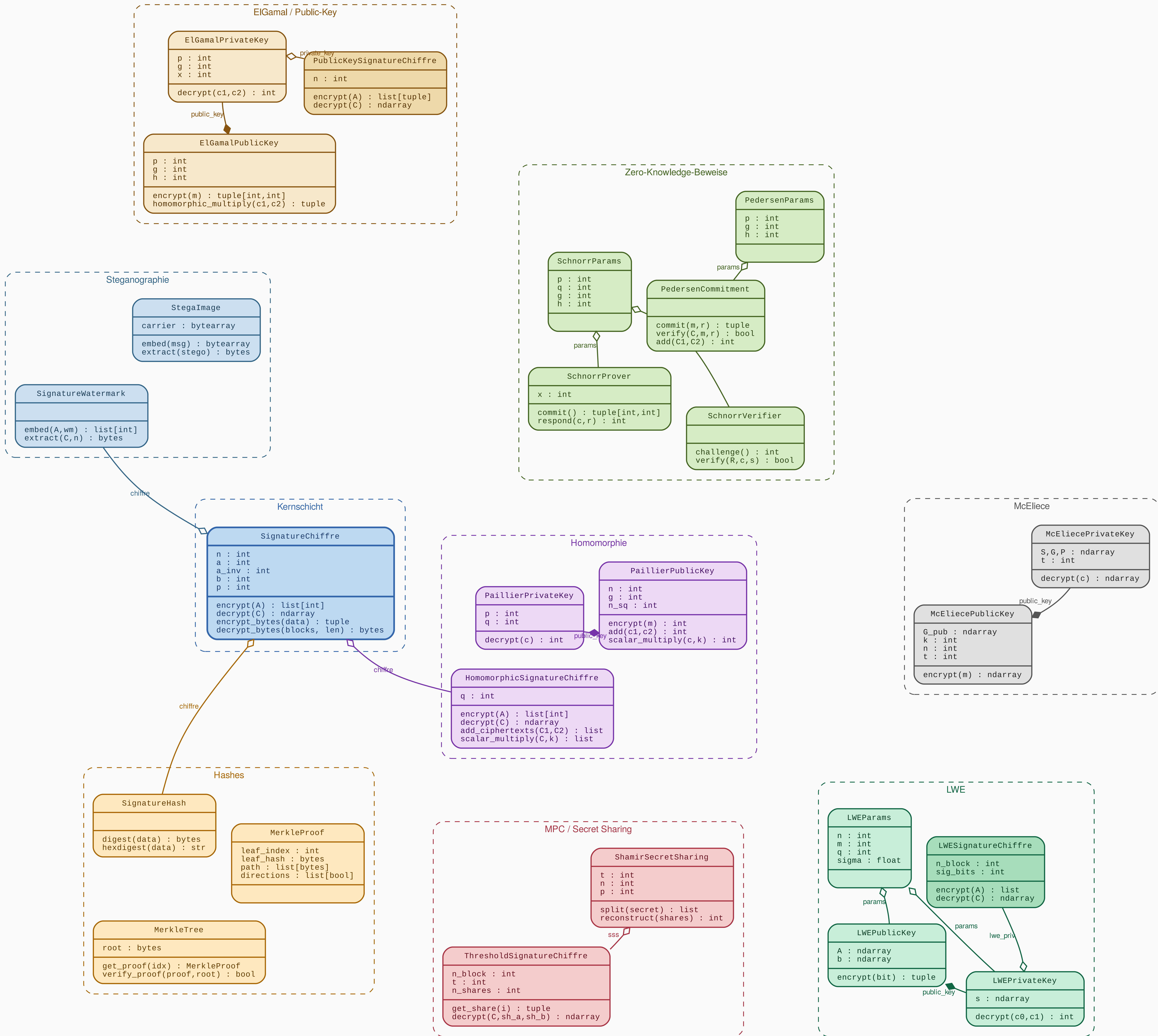
sigchiffre – Klassendiagramm ◆ Komposition ◇ Aggregation
