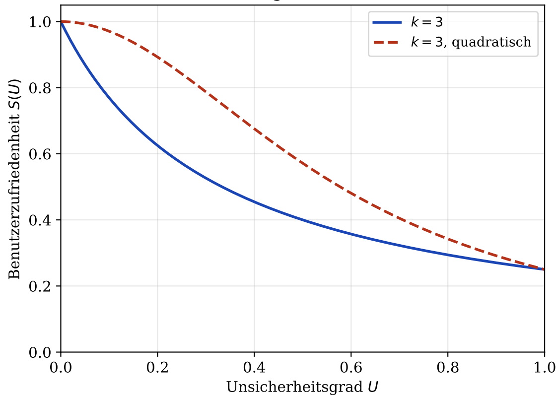
Abbildung 3b: S(U) , k = 3
