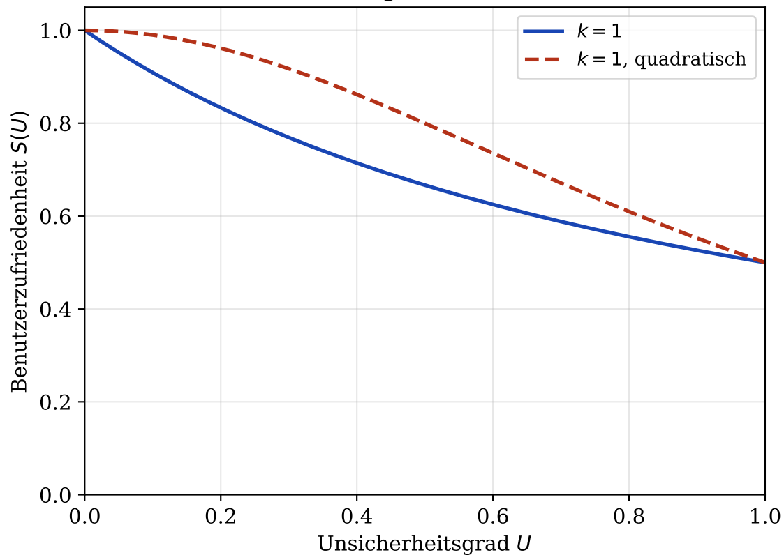
Abbildung 3a: S(U) , k = 1
