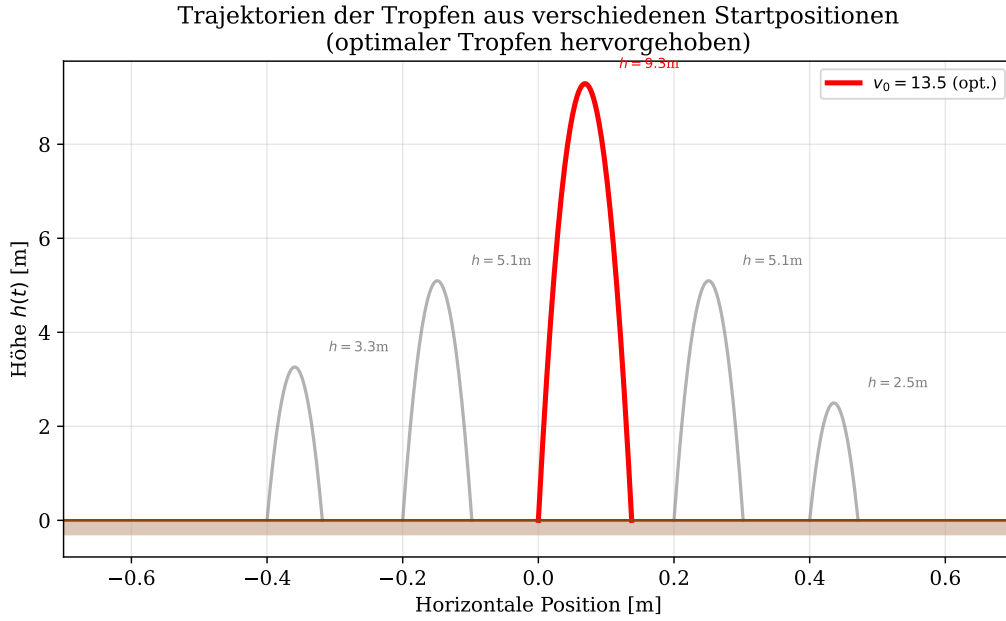
Figure 4: Trajektorien ausgewählter Tropfen aus verschiedenen radialen Startpositionen. Der optimale Tropfen (rote Kurve, v_0 = 13,5 m/s) übersteigt alle anderen klar. Die grauen Kurven zeigen Tropfen mit geringeren Startgeschwindigkeiten, die typischen Startpositionen außerhalb des optimalen Rings entsprechen. Die horizontale Achse zeigt die geringe horizontale Ablenkung durch eventuelle Seitenkomponenten; die vertikale Achse die Höhe h(t) im zeitlichen Verlauf. Der braune Bereich markiert den Kanalauslass (Bodenebene).
