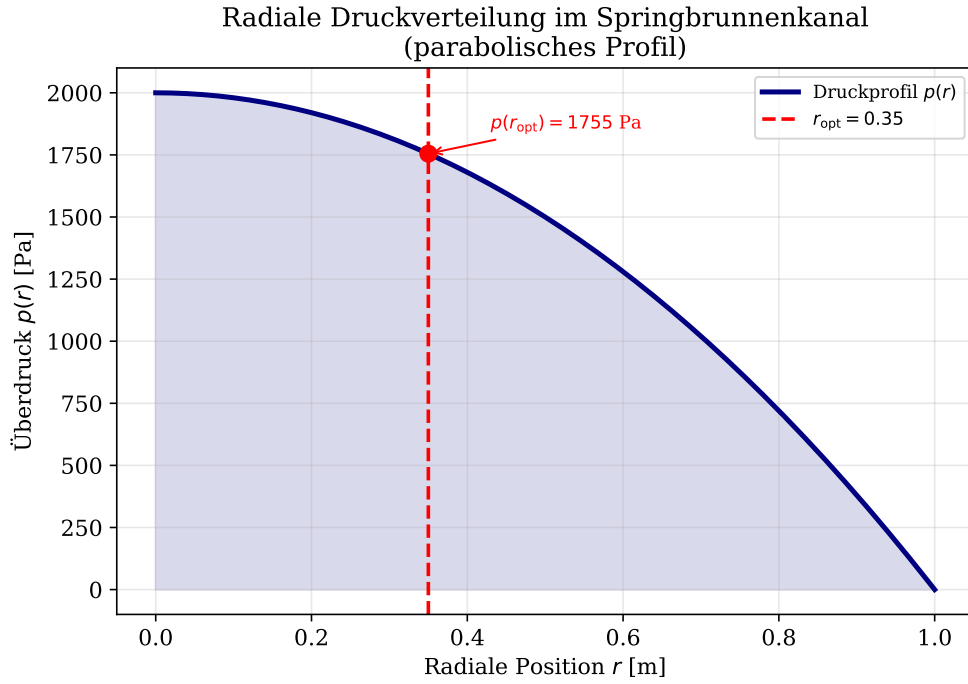
Figure 5: Radiale Druckverteilung p(r) im Kanalquerschnitt (normiert). Der Druck folgt ebenfalls einem parabolischen Profil und ist im Zentrum maximal. Die gestrichelte rote Linie markiert den optimalen Ring bei r_{\text{opt}} = 0.35 m; der rote Punkt gibt den Druckwert an dieser Position an. Der verbleibende Druckunterschied zwischen Zentrum und optimalem Ring entspricht dem “verpassten Potenzial” der Ring-Tropfen.
