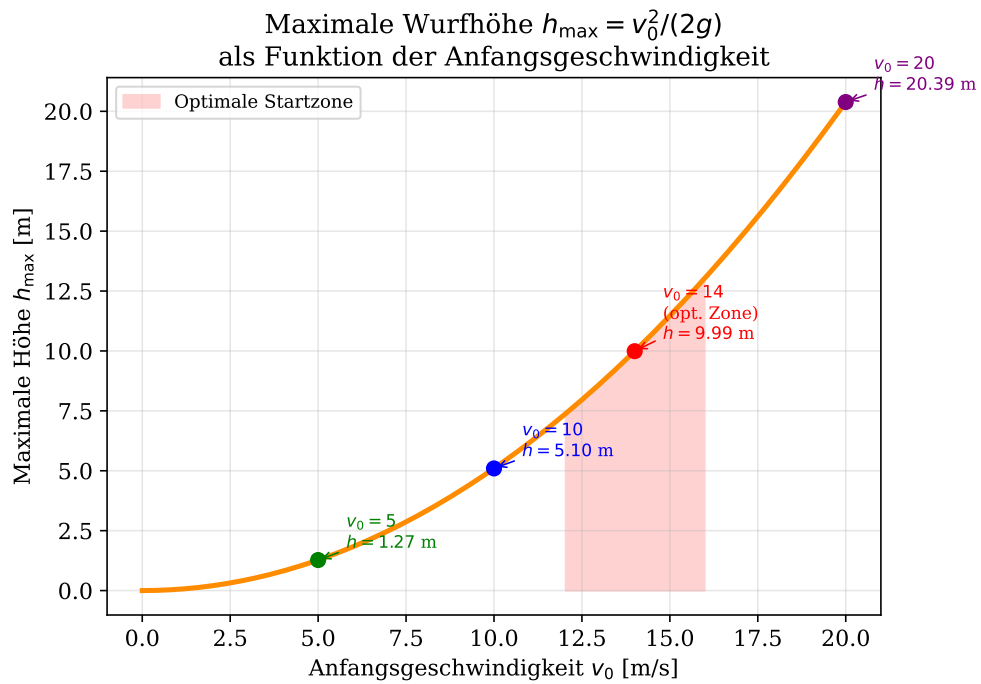
Figure 2: Maximale Aufstiegshöhe h_{\max} = v_0^2/(2g) als Funktion der Anfangsgeschwindigkeit v_0 . Die quadratische Abhängigkeit ist deutlich erkennbar: Kleine Unterschiede in v_0 führen bei höheren Geschwindigkeiten zu sehr großen Unterschieden in h_{\max} . Die rote Schattierung markiert den Bereich der optimalen Startgeschwindigkeiten ( v_0 \in [12, 16] m/s), in dem typische Springbrunnen-Tropfen operieren. Punkte markieren ausgewählte Beispiele: Der rote Punkt ( v_0 = 14 m/s, h = 10,0 m) liegt im optimalen Bereich.
