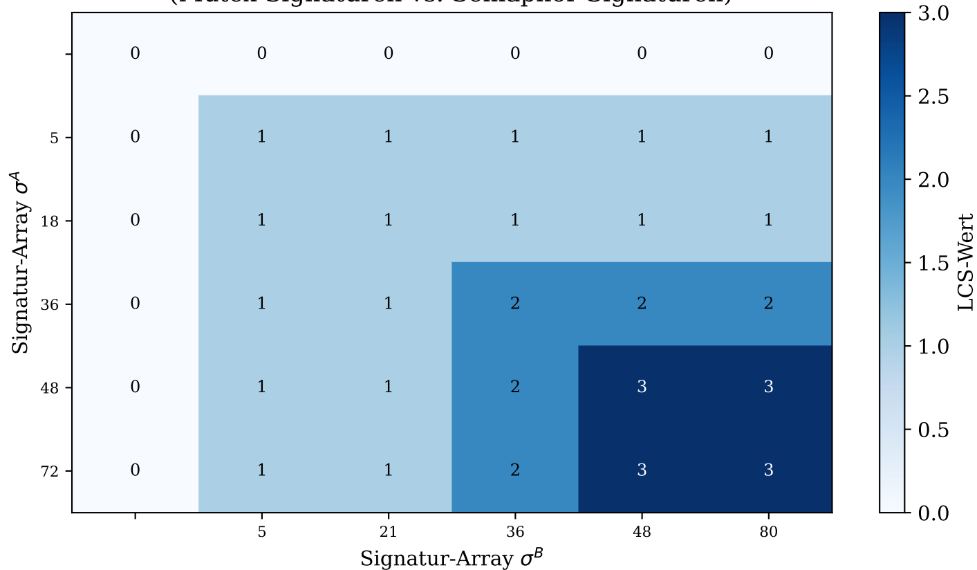
DP-Tabelle der LCS-Berechnung für zwei Signatur-Arrays (Mutex-Signaturen vs. Semaphore-Signaturen)
