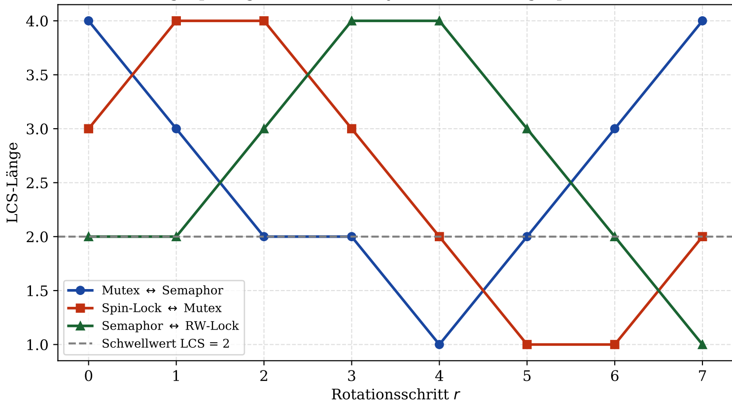
LCS-Länge über alle Rotationen (Subgraph Algorithmus auf Synchronisationsgraphen, n = 8 )
