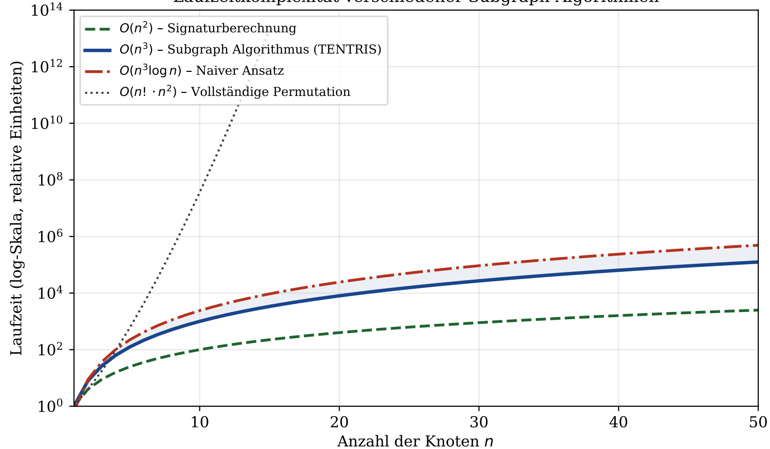
Laufzeitkomplexität verschiedener Subgraph-Algorithmen
