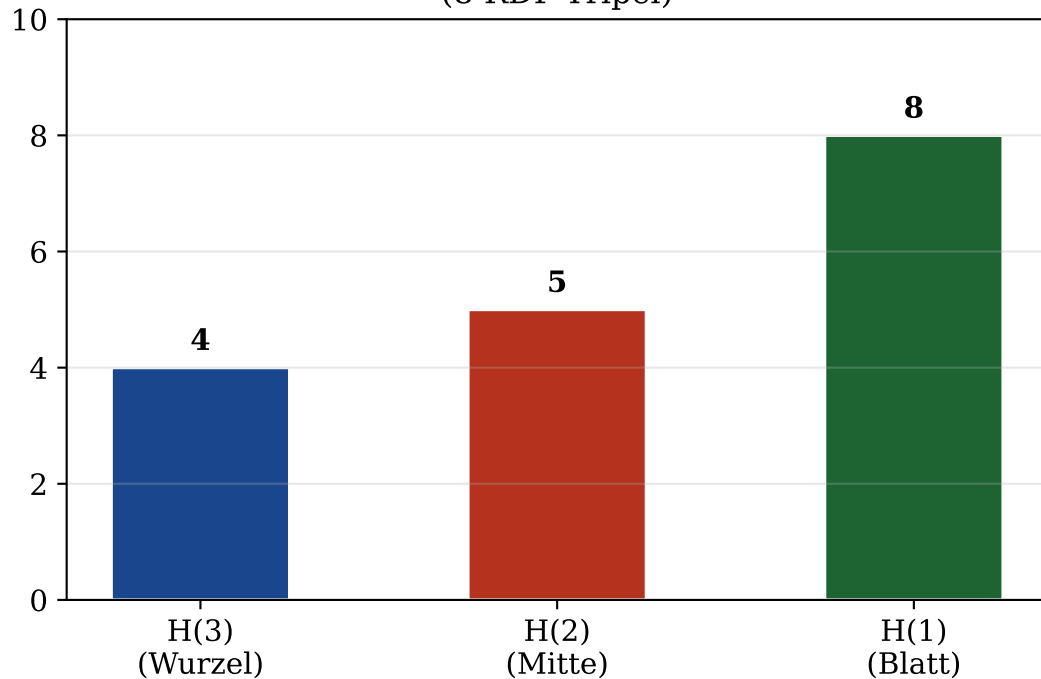
Knotenanzahl je Hypertrie-Ebene (8 RDF-Tripel)
