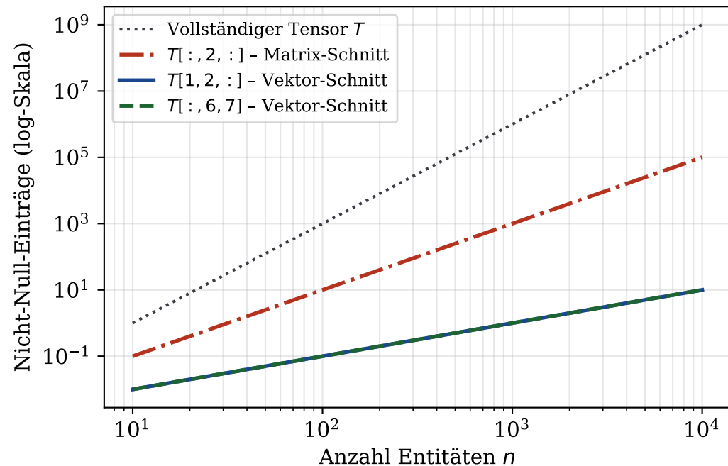
Tensor-Operandgröße in Abhängigkeit von n (Dichte = 0.1%)
