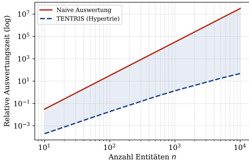
Auswertungszeit: Naive vs. TENTRIS
