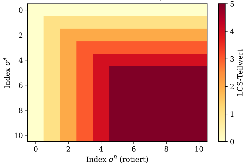
DP-Tabelle für Rotation r=0 (LCS=5)
