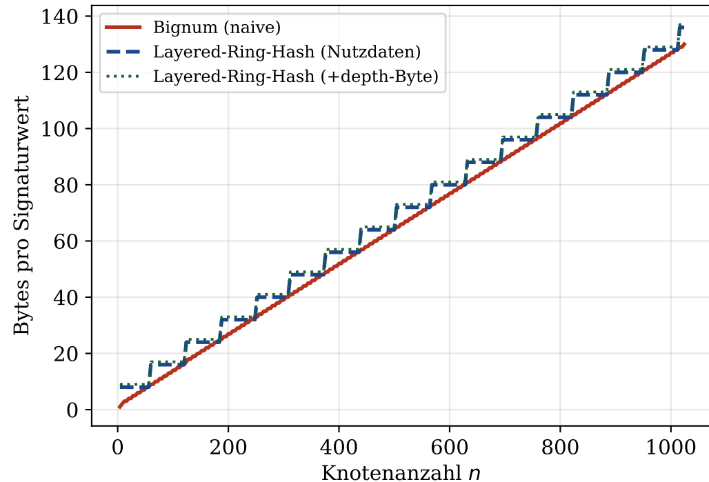
Speicherbedarf: Bignum vs. Layered-Ring-Hash
