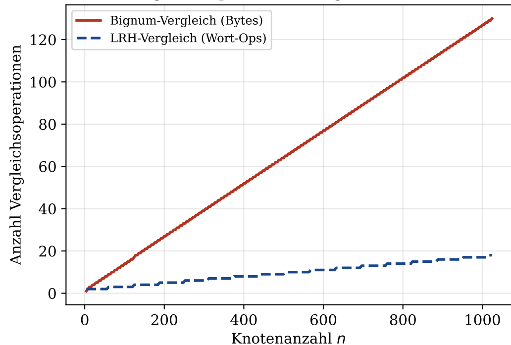
Vergleichsoperationen: Bignum vs. LRH
