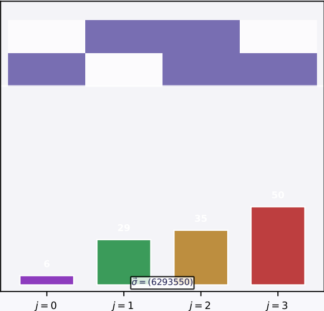
Protein-Netz (Biologie/Epidemiologie)
