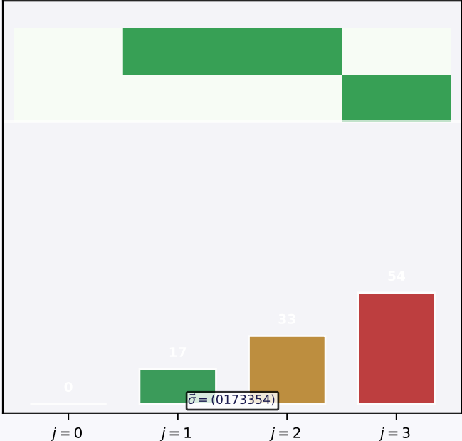
Spielgraph (Spieltheorie)
