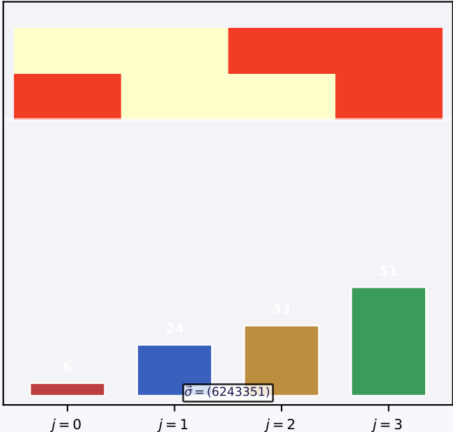
Kryptographie (Signatur-Chiffre)
