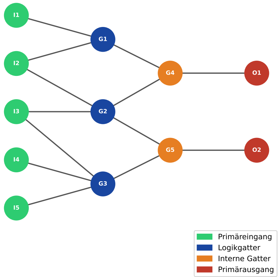
Schaltkreis als gerichteter Graph (kombinatorisches Netzwerk)
