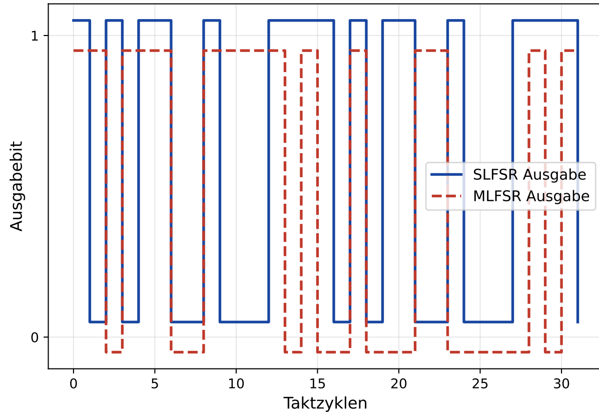
SLFSR vs. MLFSR: Ausgabesequenzen (Test-per-scan Modus, n=4)
