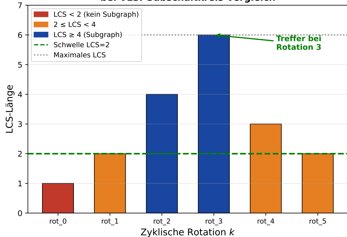
Subgraph-Algorithmus: LCS pro Rotation bei VLSI-Subschaltkreis-Vergleich
