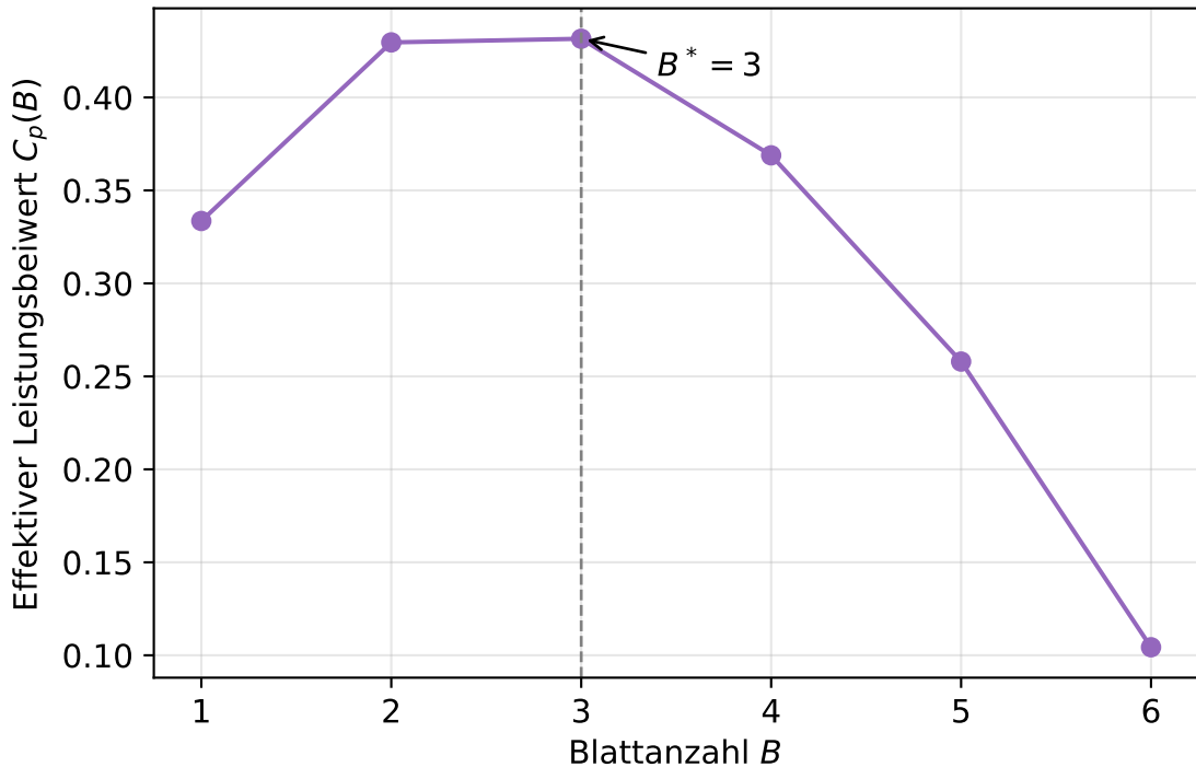
Leistungsbeiwert in Abhängigkeit der Blattanzahl
