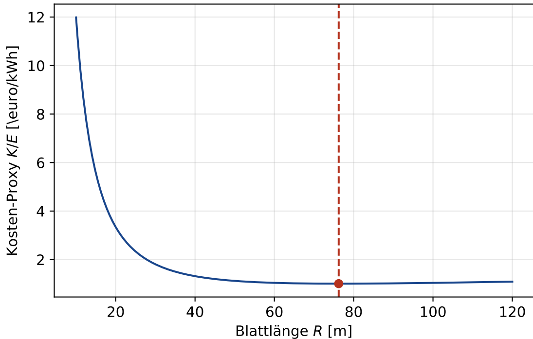
Kosten-Ertrags-Verhältnis vs. Blattlänge ( H = 100 m, Land)
