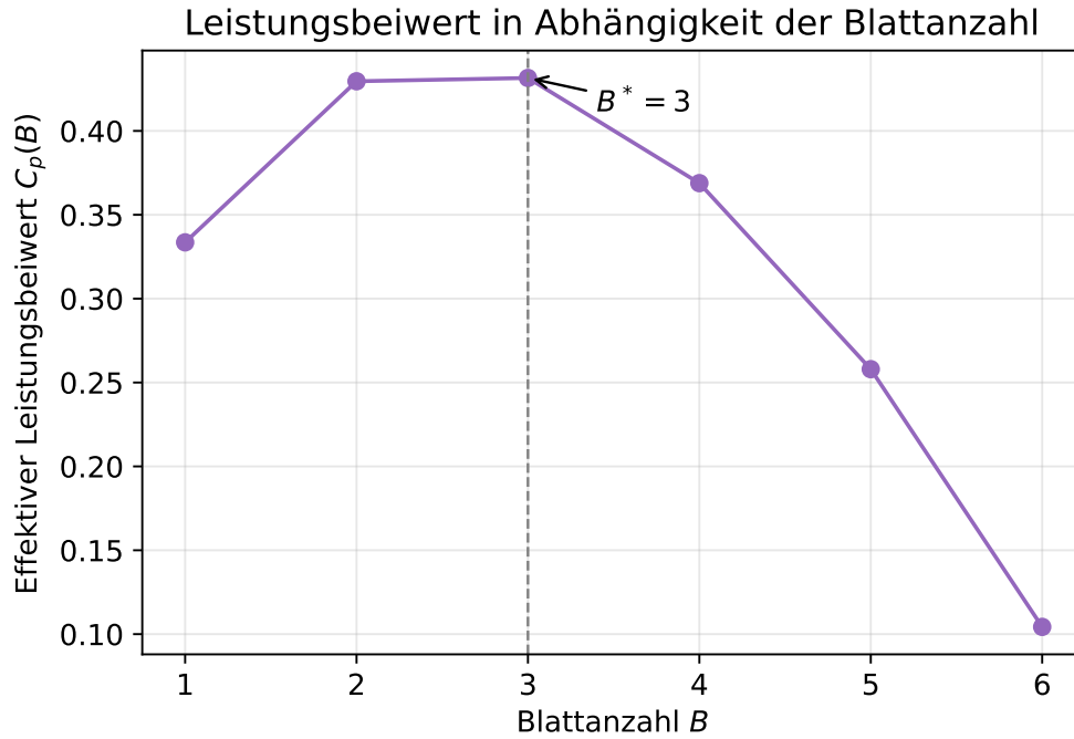
Figure 5: Effektiver Leistungsbeiwert C_p(B) nach Definition 5. Das Maximum liegt bei B^* = 3 ; sowohl der Ein-Blatt- als auch höhere Mehrblatt-Konfigurationen ( B \geq 4 ) liefern aufgrund von Reibungs- und Interaktionsverlusten einen geringeren effektiven Leistungsbeiwert.
