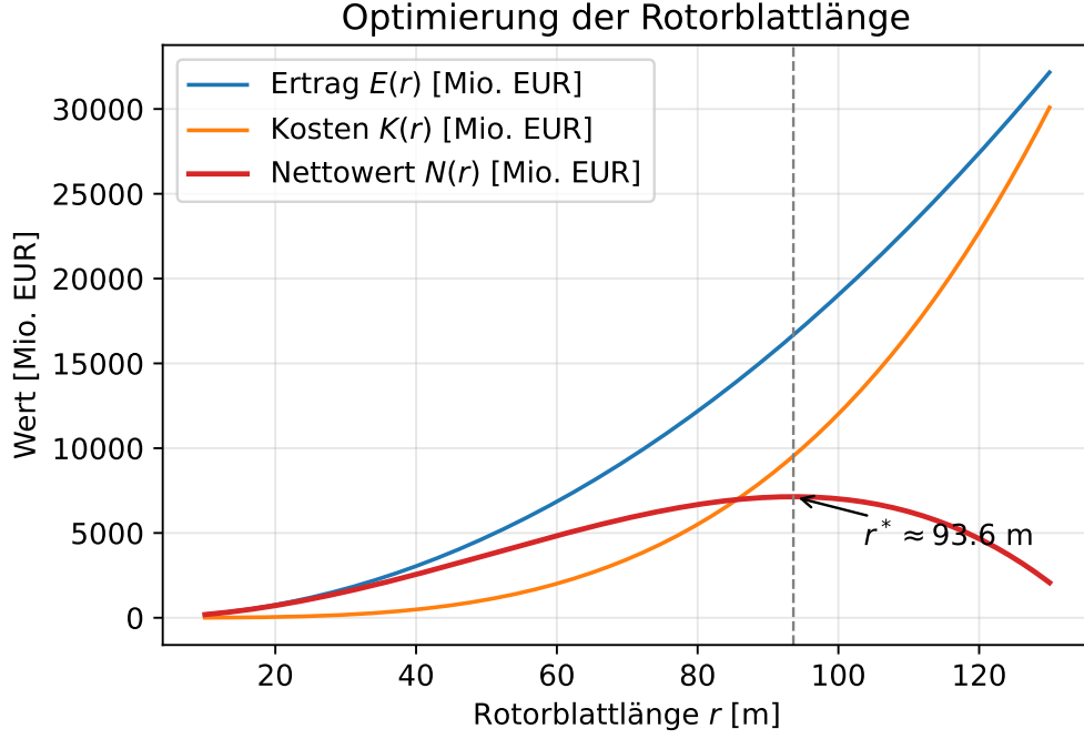
Figure 4: Ertrag E(r) \propto r^2 , Kosten K(r) = \kappa_1 r^{3,5} + \kappa_2 r^{2,5} und Nettowert N(r) = E(r) - K(r) . Das Optimum bei r^* \approx 93,6 m markiert den Punkt, an dem die Grenzkosten eines weiteren Längenmeters den Grenzertrag übersteigen.
