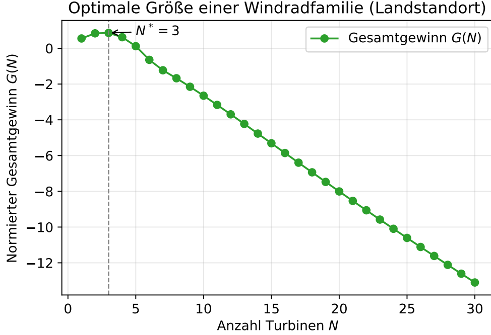
Figure 7: Normierter Gesamtgewinn G(N) unter Berücksichtigung von Flächen-/Pachtkosten pro Anlage. Das Maximum bei N^* = 3 markiert die Stelle, an der der Grenzgewinn einer zusätzlichen, durch Nachlaufeffekte geschwächten Turbine die zugehörigen Flächenkosten nicht mehr deckt.
