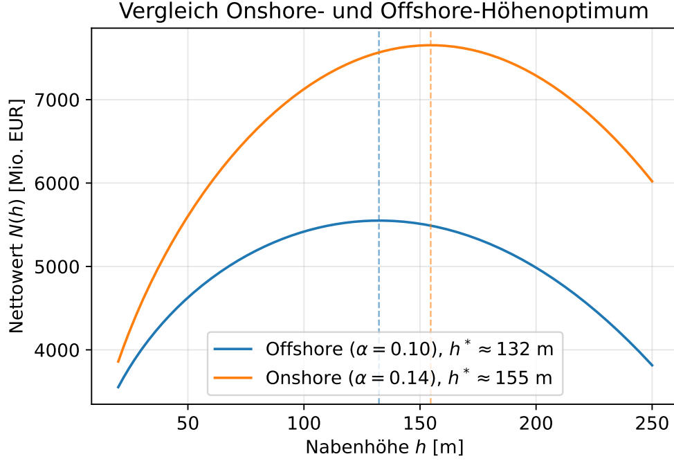
Figure 3: Vergleich des Nettowert-Optimums für Onshore- ( \alpha = 0,14 ) und Offshore-Standorte ( \alpha = 0,10 ) bei sonst identischen Kostenparametern. Der geringere Rauigkeitsexponent Offshore führt zu einem etwas niedrigeren optimalen h^* , da der Mehrertrag durch zusätzliche Höhe geringer ausfällt – in der Praxis wird dies jedoch häufig durch andere Faktoren (z. B. größere zulässige Rotordurchmesser durch fehlende Transportbeschränkungen) überlagert.
