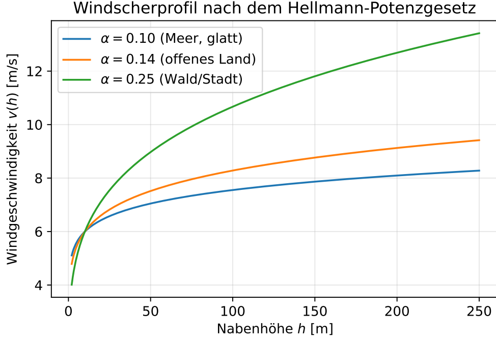
Figure 1: Windscherprofil v(h) nach dem Hellmann-Potenzgesetz für drei Rauigkeitsklassen. Mit zunehmendem \alpha (rauere Oberfläche) steigt die Windgeschwindigkeit mit der Höhe stärker an, was den Anreiz für höhere Türme erhöht.
