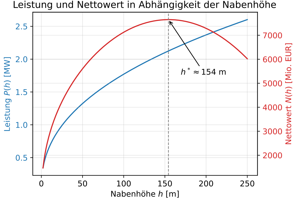
Figure 2: Leistung P(h) (links, blau) und Nettowert N(h) = E(h) - K(h) (rechts, rot) über der Nabenhöhe für \alpha = 0,14 . Während P(h) monoton wächst, besitzt N(h) ein eindeutiges inneres Maximum bei h^* \approx 154 m, das aus dem Schnittpunkt des sublinearen Ertragswachstums ( h^{3\alpha} , 3\alpha = 0,42 ) mit dem superlinearen Kostenwachstum ( h^{2,6} ) resultiert.
