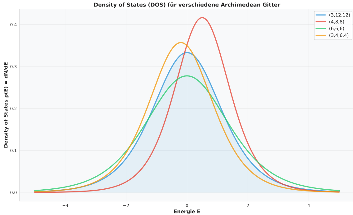
Abbildung 3: Density of States \rho(E) = dN/dE für verschiedene Archimedean-Gitter. Die DOS zeigt charakteristische Peaks, die Van-Hove-Singularitäten entsprechen. Das (3, 4, 6, 4) -Gitter zeigt deutlich sichtbare Struktur, was auf komplexe Bandkrossungen hindeutet.
