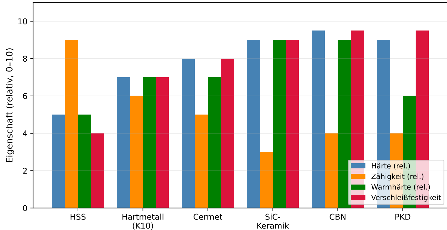
Vergleich mechanischer Eigenschaften von Schneidstoffklassen
