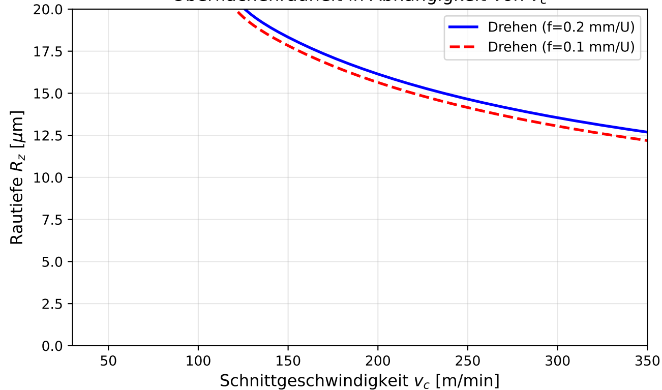
Oberflächenrauheit in Abhängigkeit von v_c
