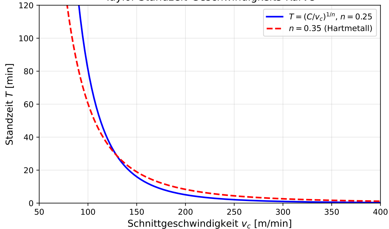
Taylor-Standzeit-Geschwindigkeits-Kurve
