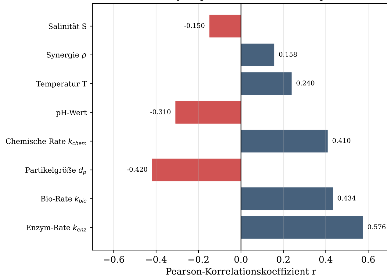
Sensitivitätsanalyse: Tornado-Diagramm (Einfluss auf synergistische Neutralisierungseffizienz)
