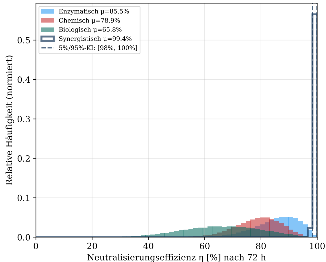
Monte-Carlo-Verteilung der Neutralisierungseffizienz (n = 50,000 Simulationen)
