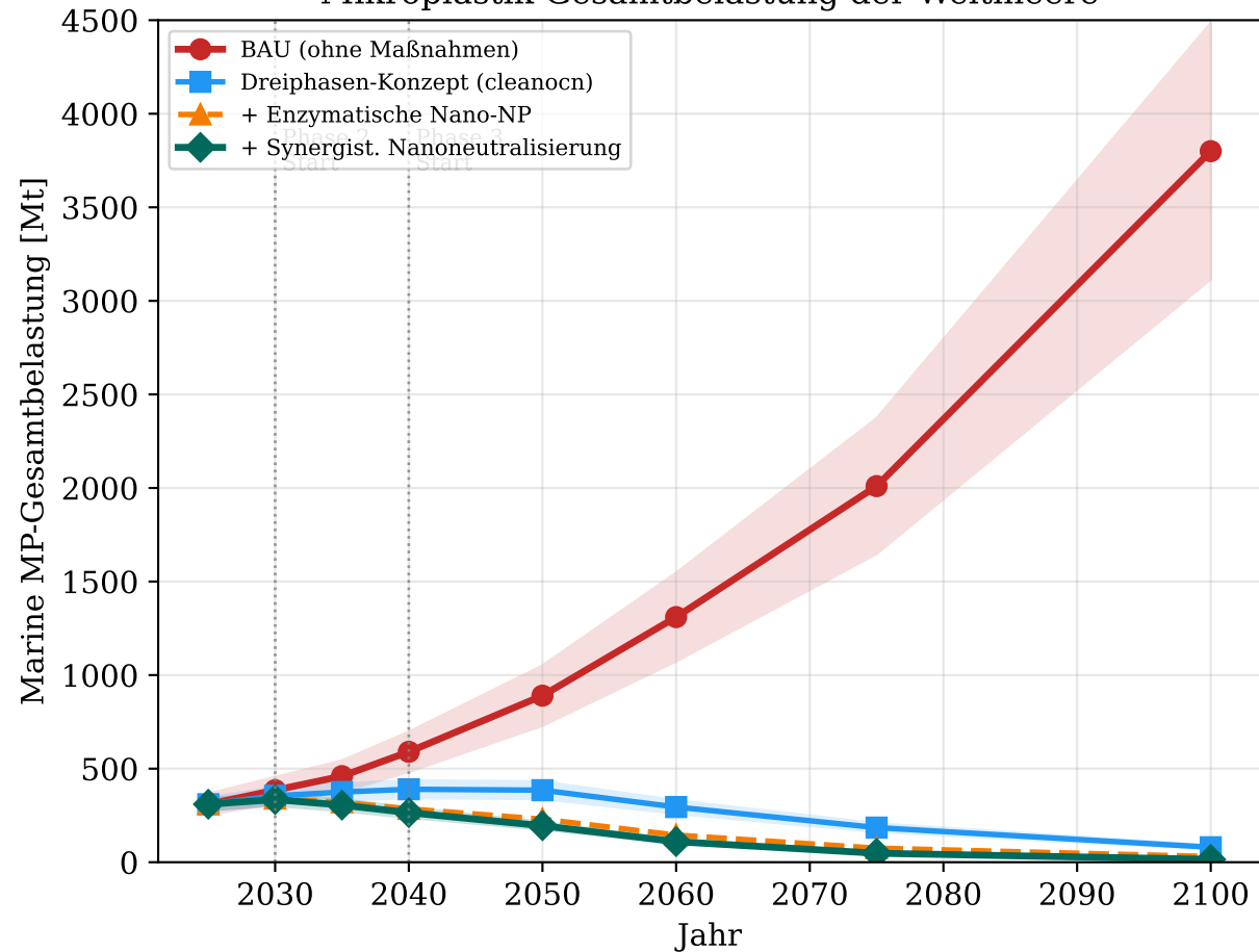
Szenarioprognose 2025-2100: Mikroplastik-Gesamtbelastung der Weltmeere
