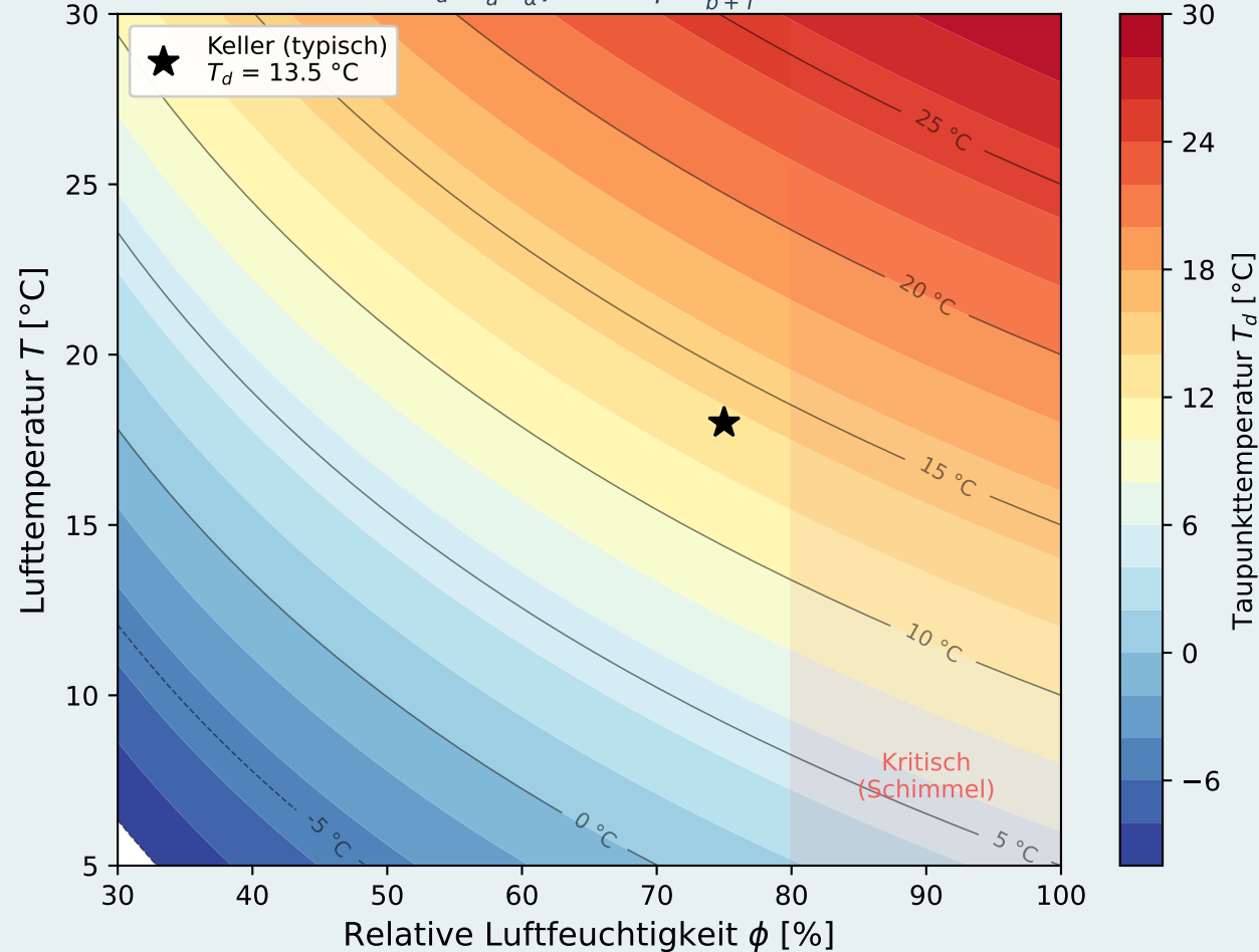
Taupunkttemperatur (Magnus-Formel)
