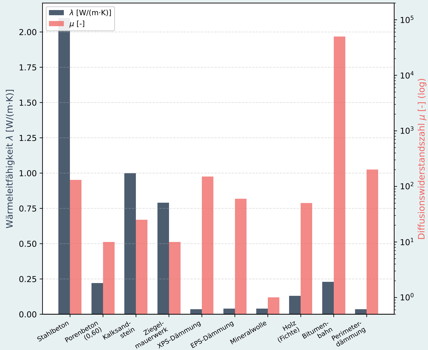
Wärmeleitfähigkeit und Diffusionswiderstand von Baustoffen (DIN EN ISO 10456)
