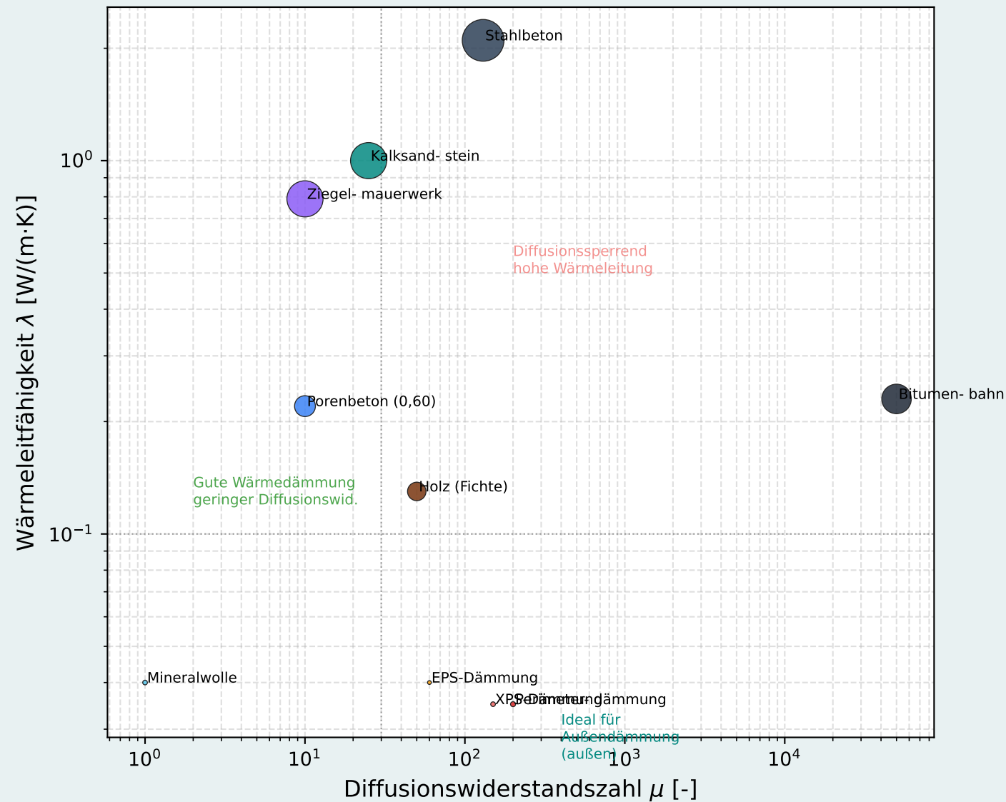
Baustoffauswahl: \lambda vs. \mu (Punktgröße \propto Rohdichte \rho )
