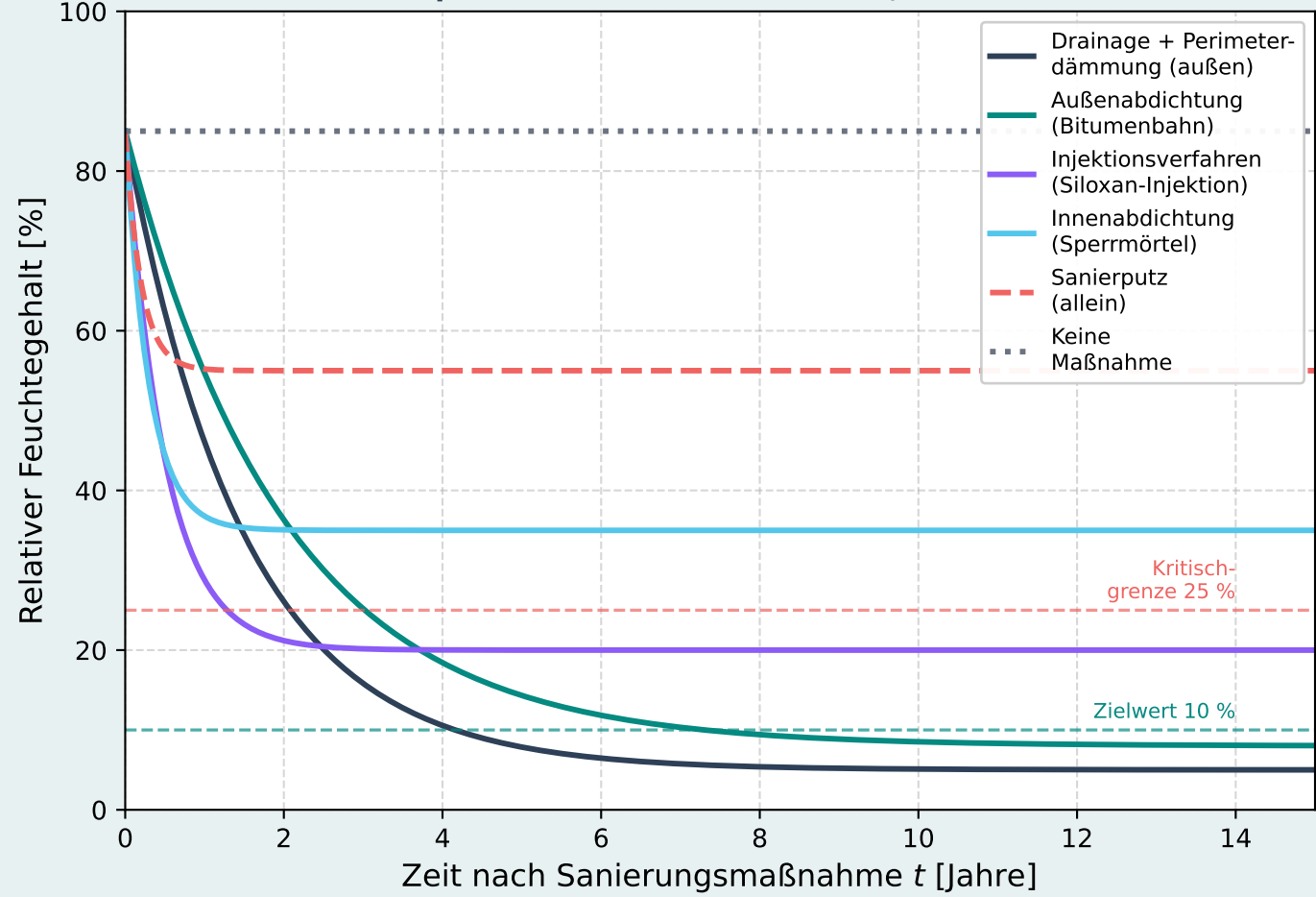
Feuchtegehalt nach Sanierungsmaßnahmen (Exponentialmodell u(t) = u_{\infty} + (u_0 - u_{\infty})e^{-t/\tau} )
