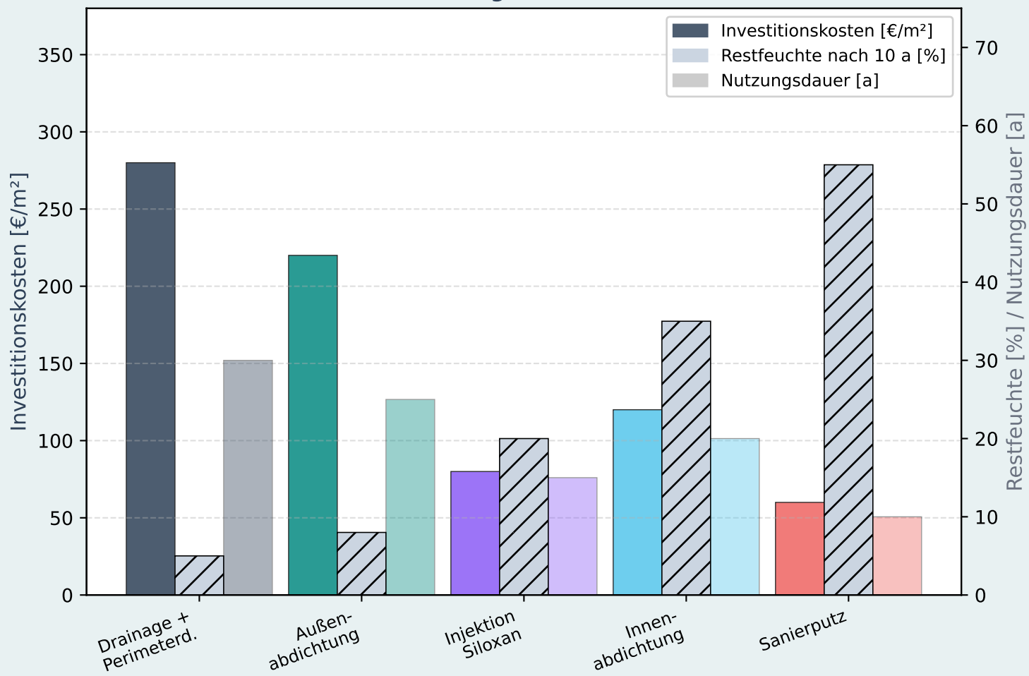
Wirtschaftlichkeitsvergleich Sanierungsmaßnahmen
