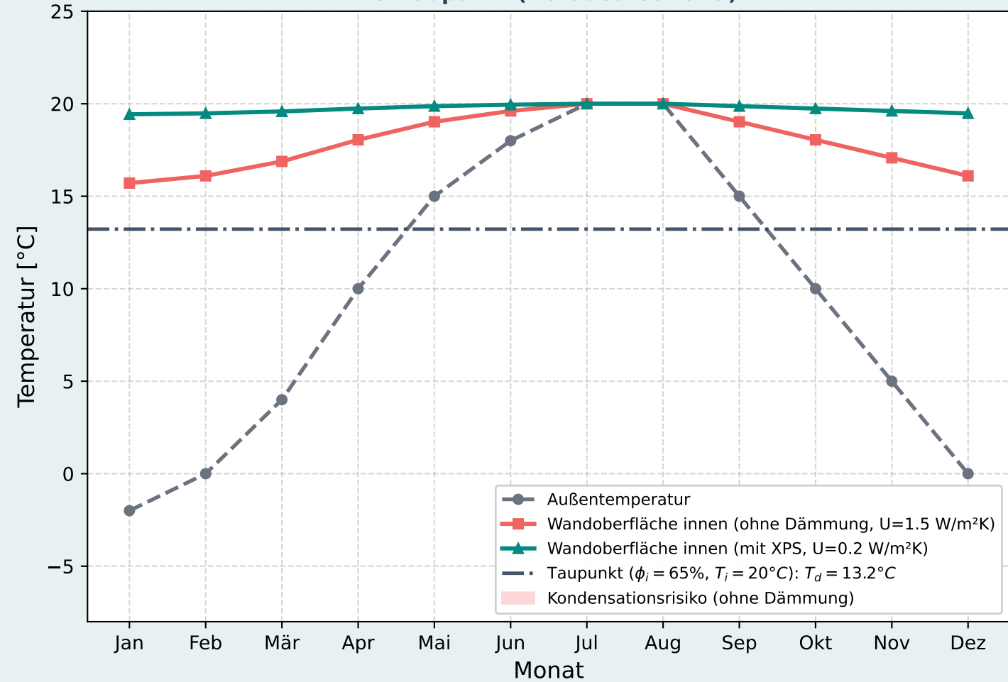
Jahresgang Wandoberflächentemperatur vs. Taupunkt (Norddeutschland)
