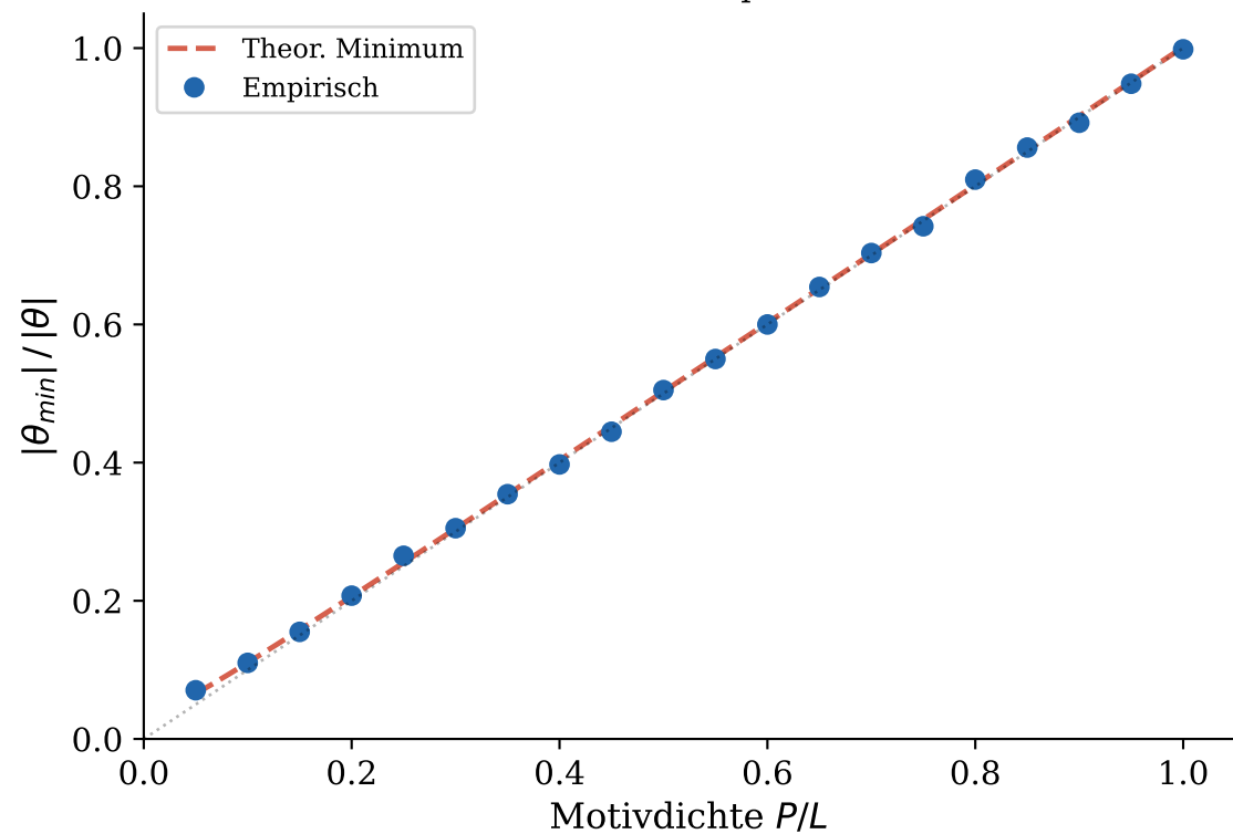
Parameterkompression
