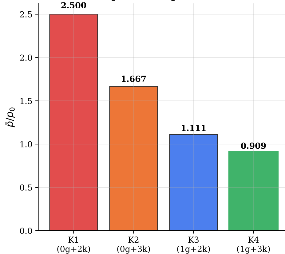
Mittlere Flächenpressung (niedriger = weniger Verschleiß)
