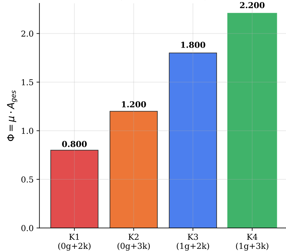
Gütekriterium Bremskraft/Verschleiß (höher = besser)
