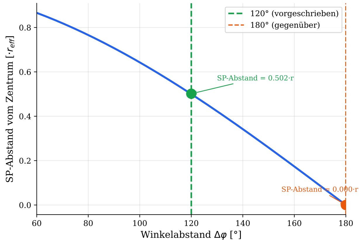
Schwerpunktlage der 2 kl. Klötze vs. Winkelabstand
