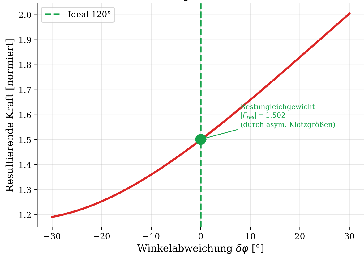
Robustheit K3 bei Montagetoleranzen
