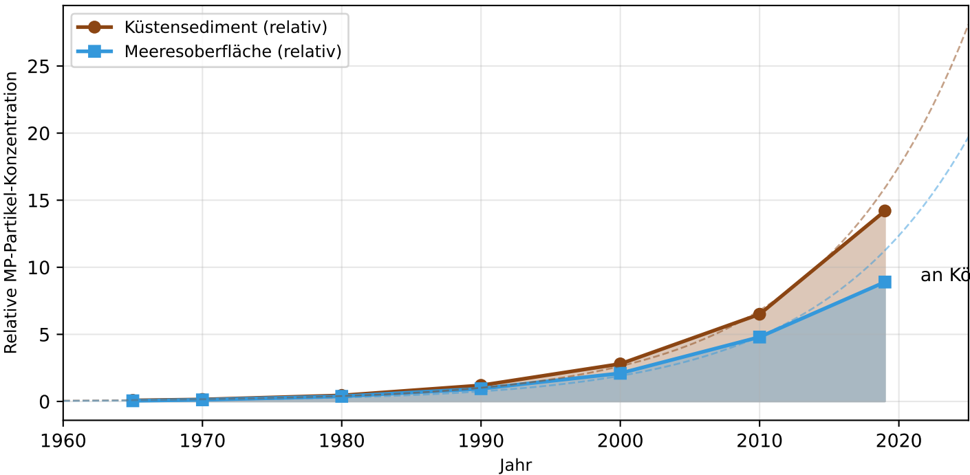
C) Multidekadische Zunahme von MP in Küstensedimenten und Meeresoberfläche (Brandon et al. 2019; Hale et al. 2020 - normierte Einheiten)
