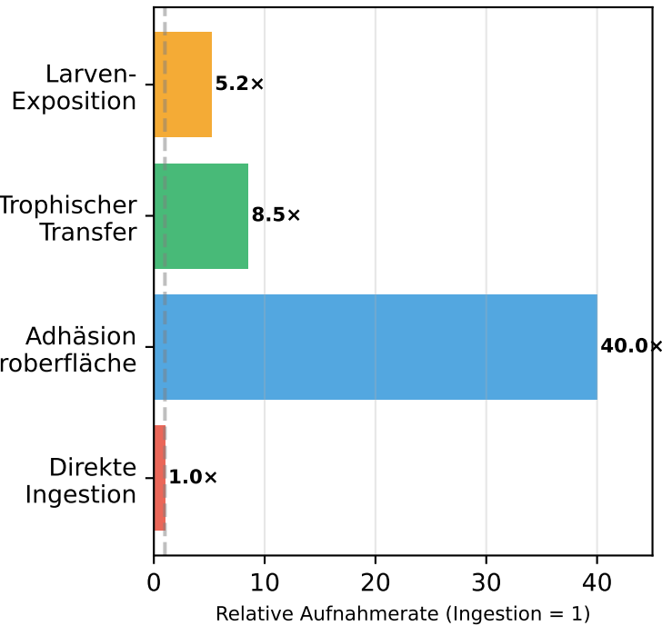
D) Relative Aufnahmeraten von MP durch Korallen (Martin et al. 2019)
