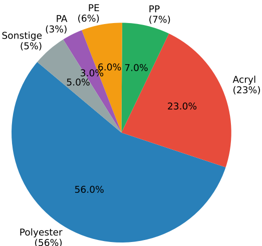
B) Polymer-Typen an weltweiten Strandstandorten (Browne et al. 2011, n=18 Kontinente)
