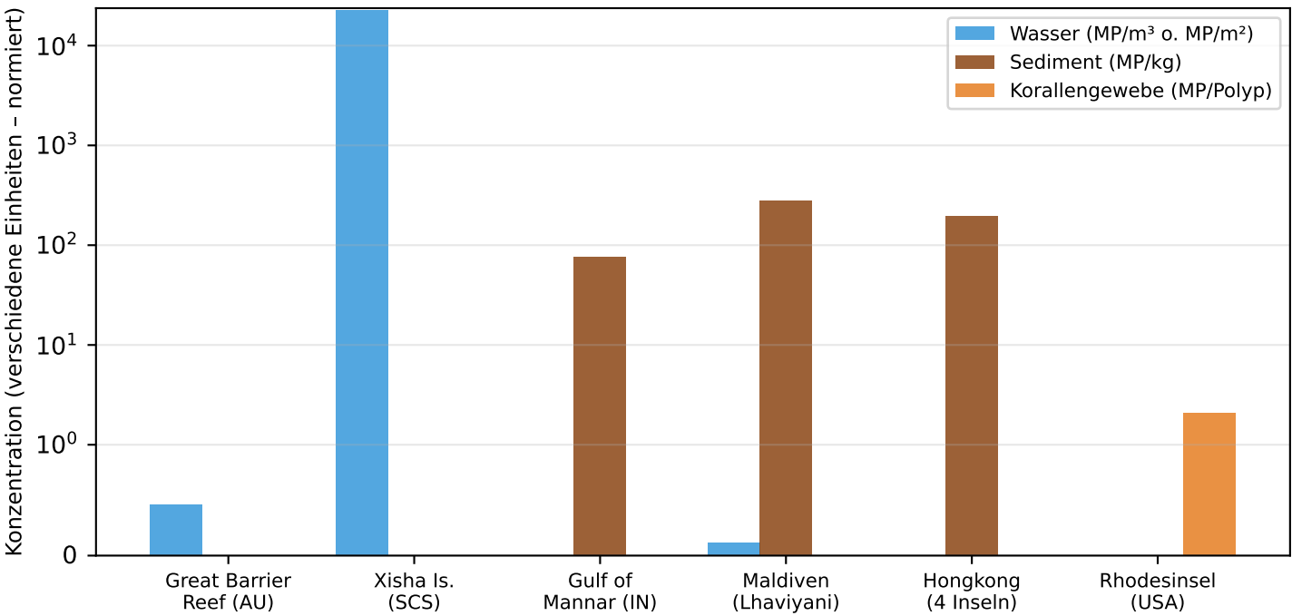
A) MP-Konzentrationen in Korallenriffen nach Meeresgebiet (Anmerkung: Einheiten variieren, Darstellung normiert für Vergleichbarkeit)
