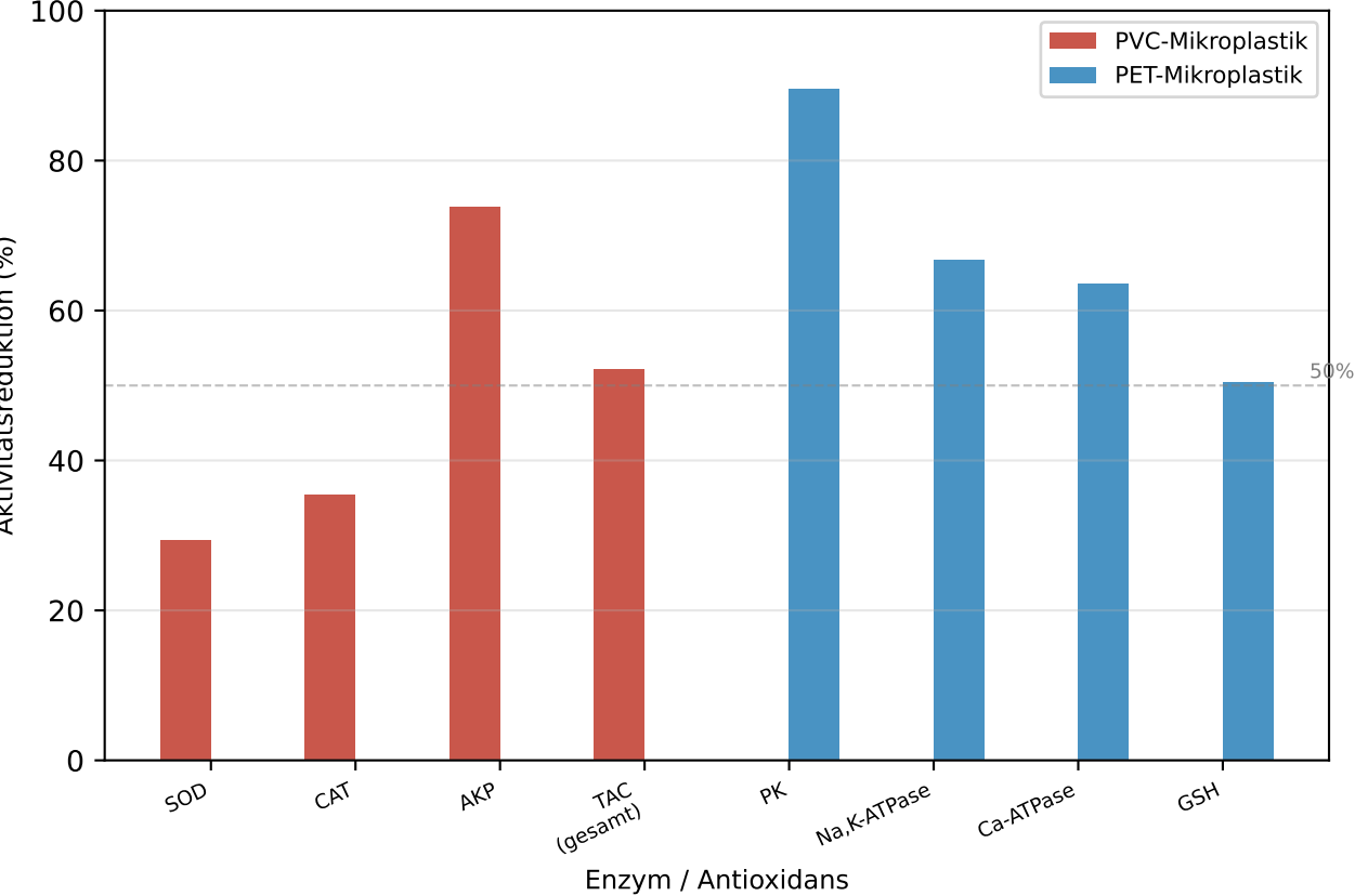
A) Reduktion enzymatischer Aktivitäten ( Tubastrea aurea )
