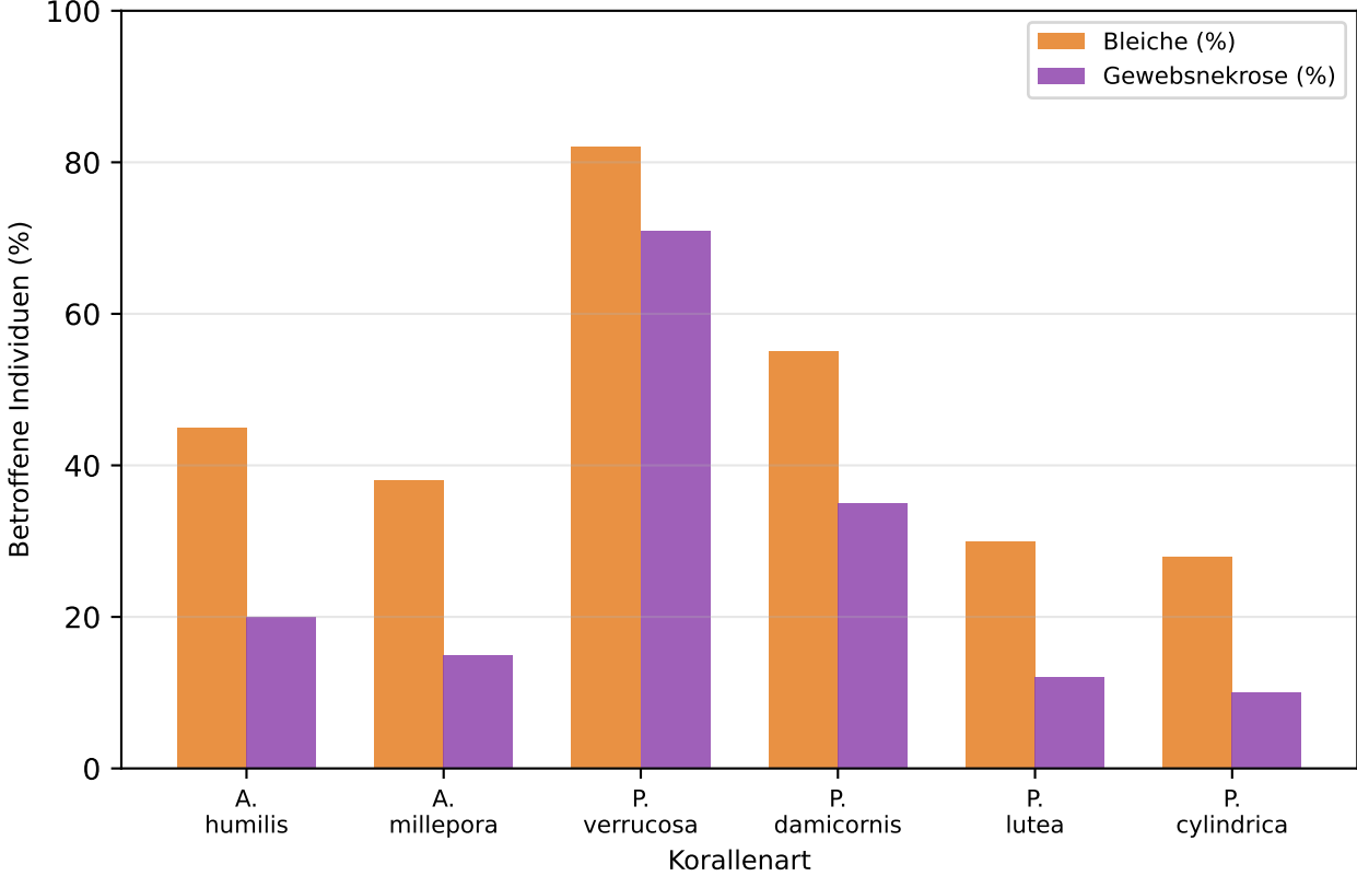
B) Bleiche und Nekrose nach MP-Exposition (3.799 ± 546 MP/L, 28 Tage)
