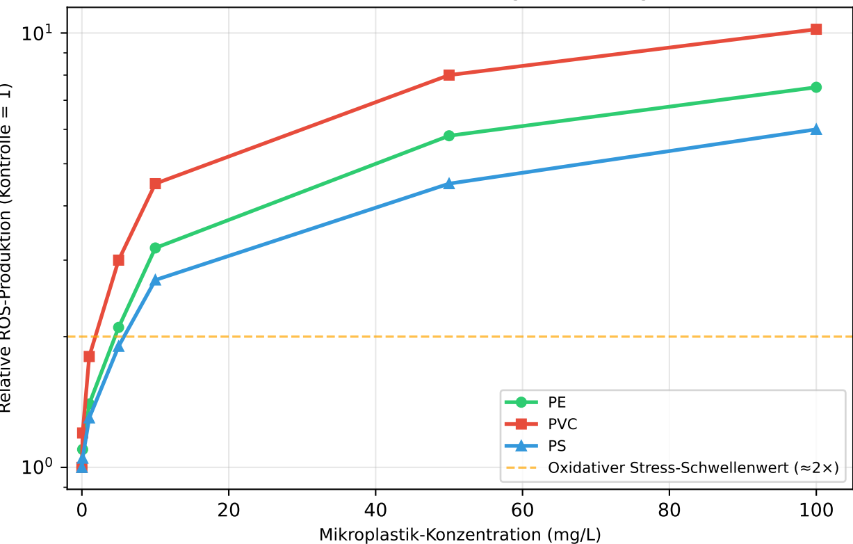
C) ROS-Produktionskinetik bei MP-Exposition (Konzentrations-Wirkungs-Beziehung)
