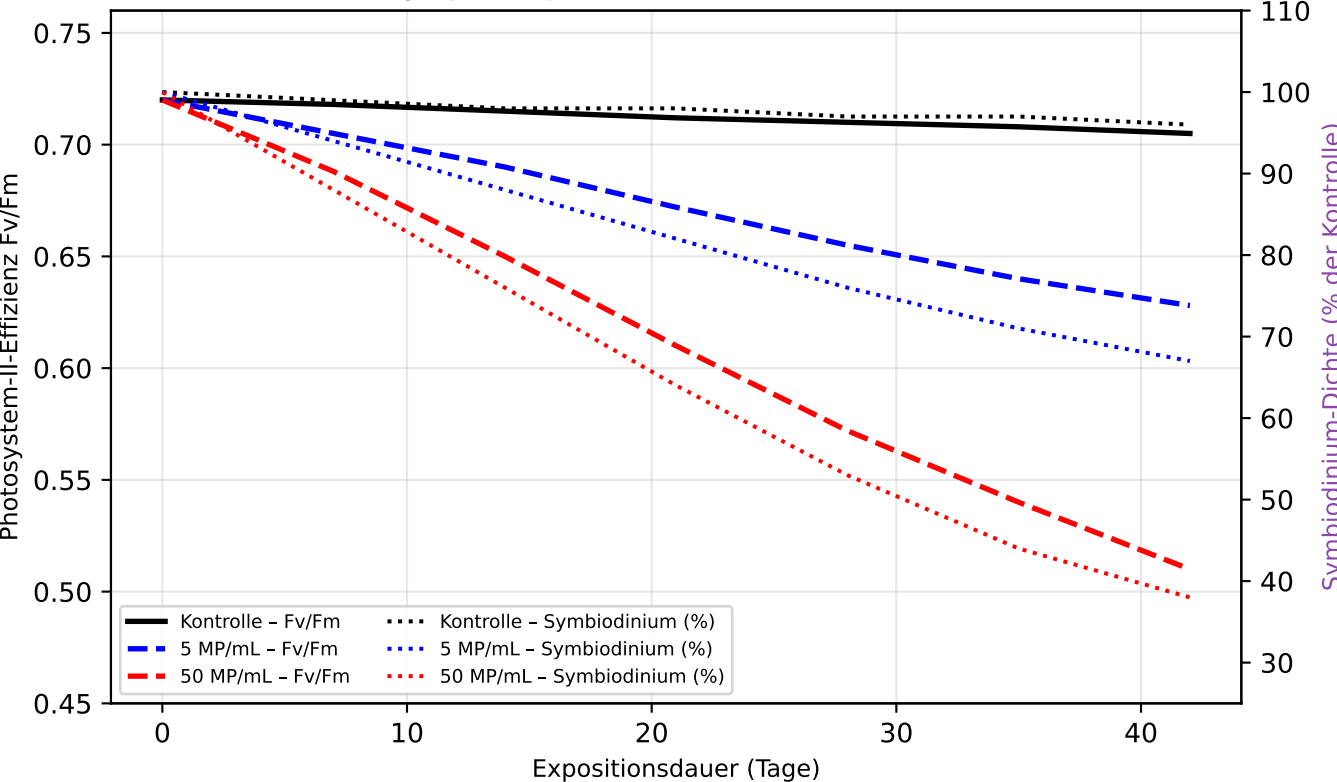
D) Photosynthese-Effizienz und Symbiodinium-Dichte ( Stylophora pistillata , Lanctôt et al. 2020)
