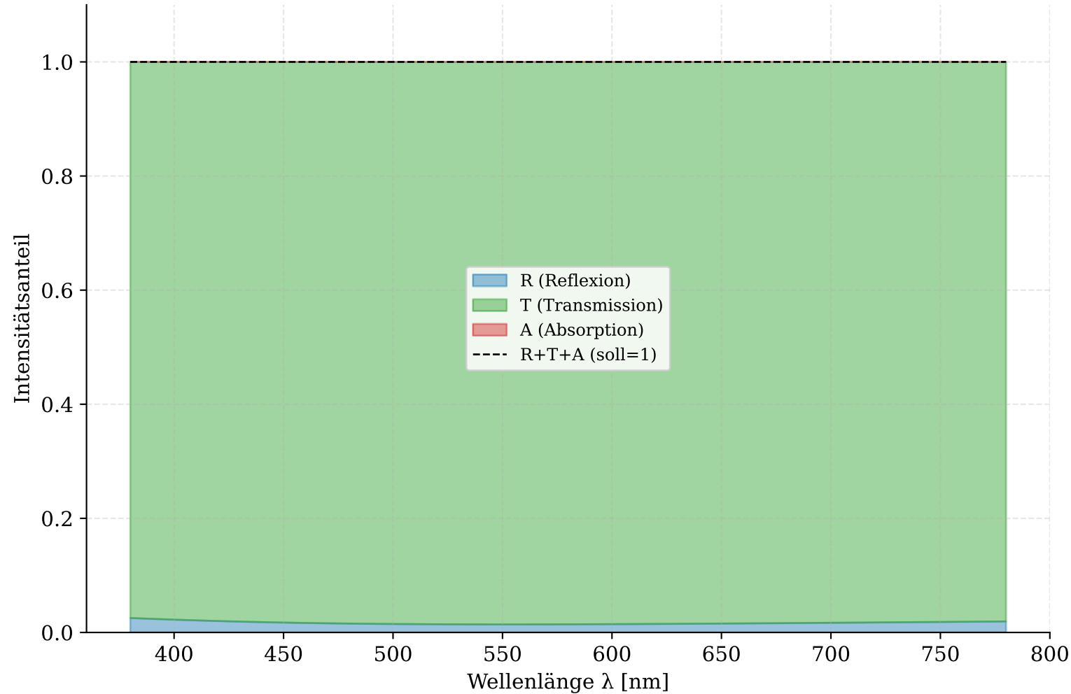
MgF 2 -Antireflexschicht (d=100 nm, n=1.38)
