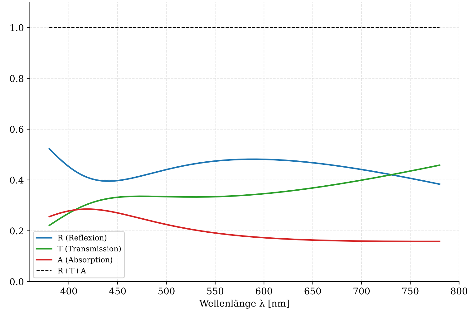
PDMS (200 nm) + Au-Spiegel (30 nm) auf SiO 2
