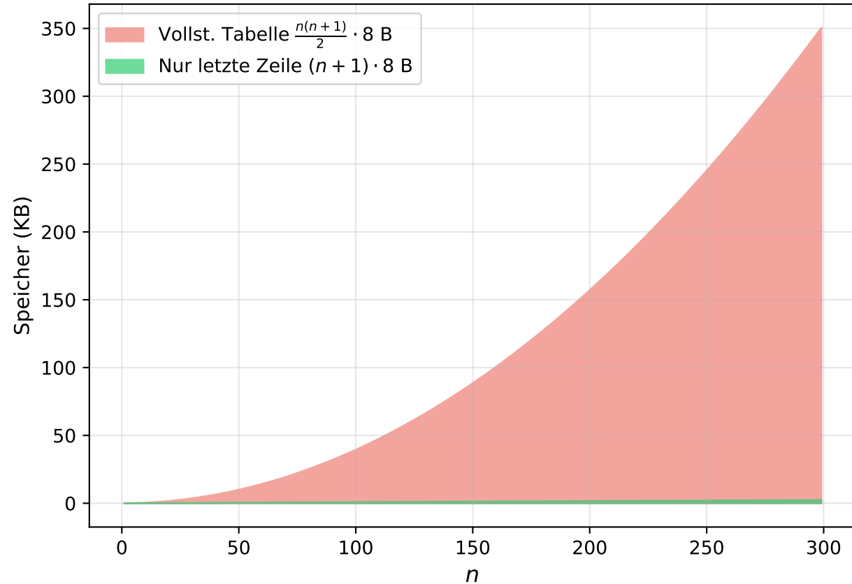
Speicherbedarf: Tabelle vs. Zeilenansatz
