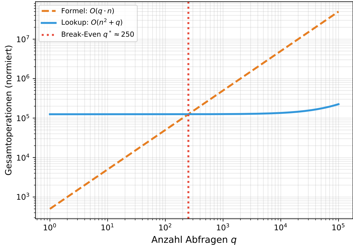
Amortisierte Analyse ( n = 500 )
