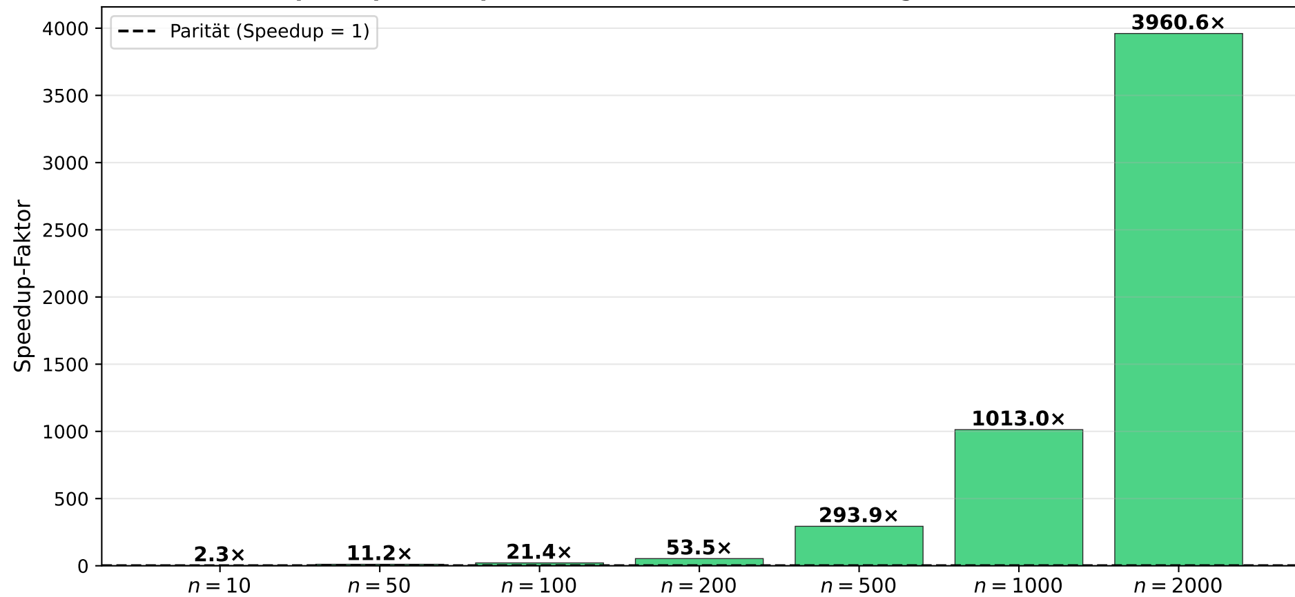
Speedup: Lookup vs. Fakultätsformel (5000 Abfragen nach Aufbau)
