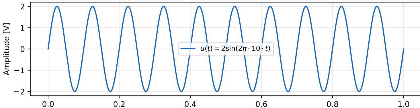
Eingangssignal: SinusoidalSource
