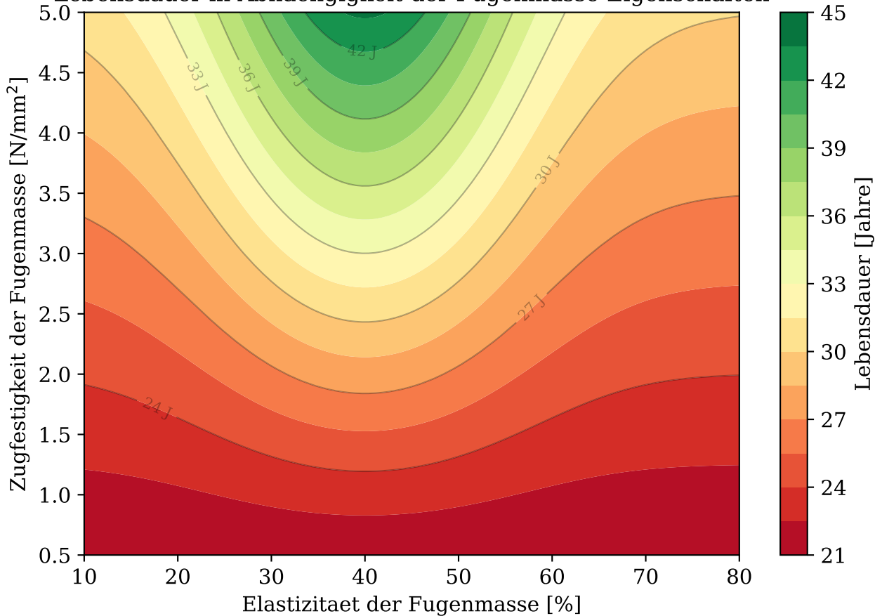
Lebensdauer in Abhaengigkeit der Fugenmasse-Eigenschaften
