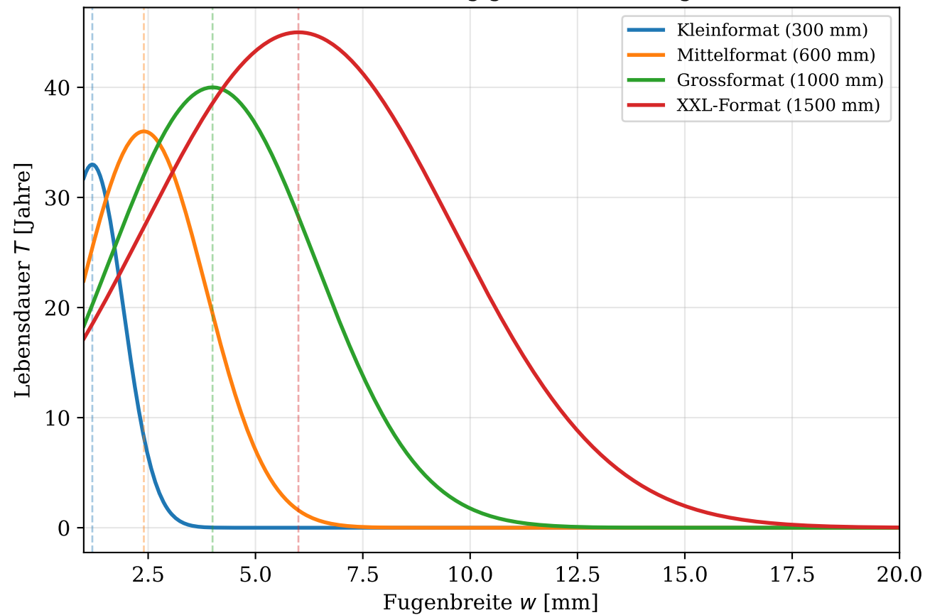
Lebensdauer in Abhaengigkeit von der Fugenbreite
